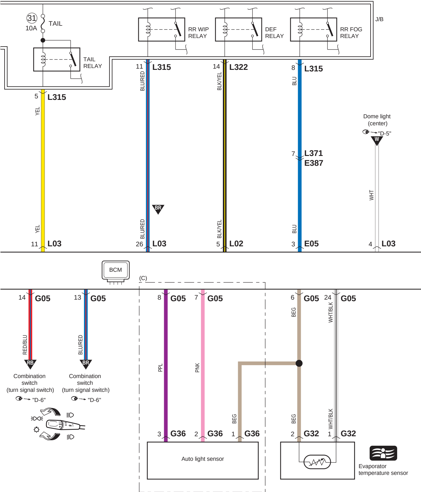
A-8-2 Diagrama del circuito del sistema de control de la carrocería (con sistema de arranque por pulsación del motor)
