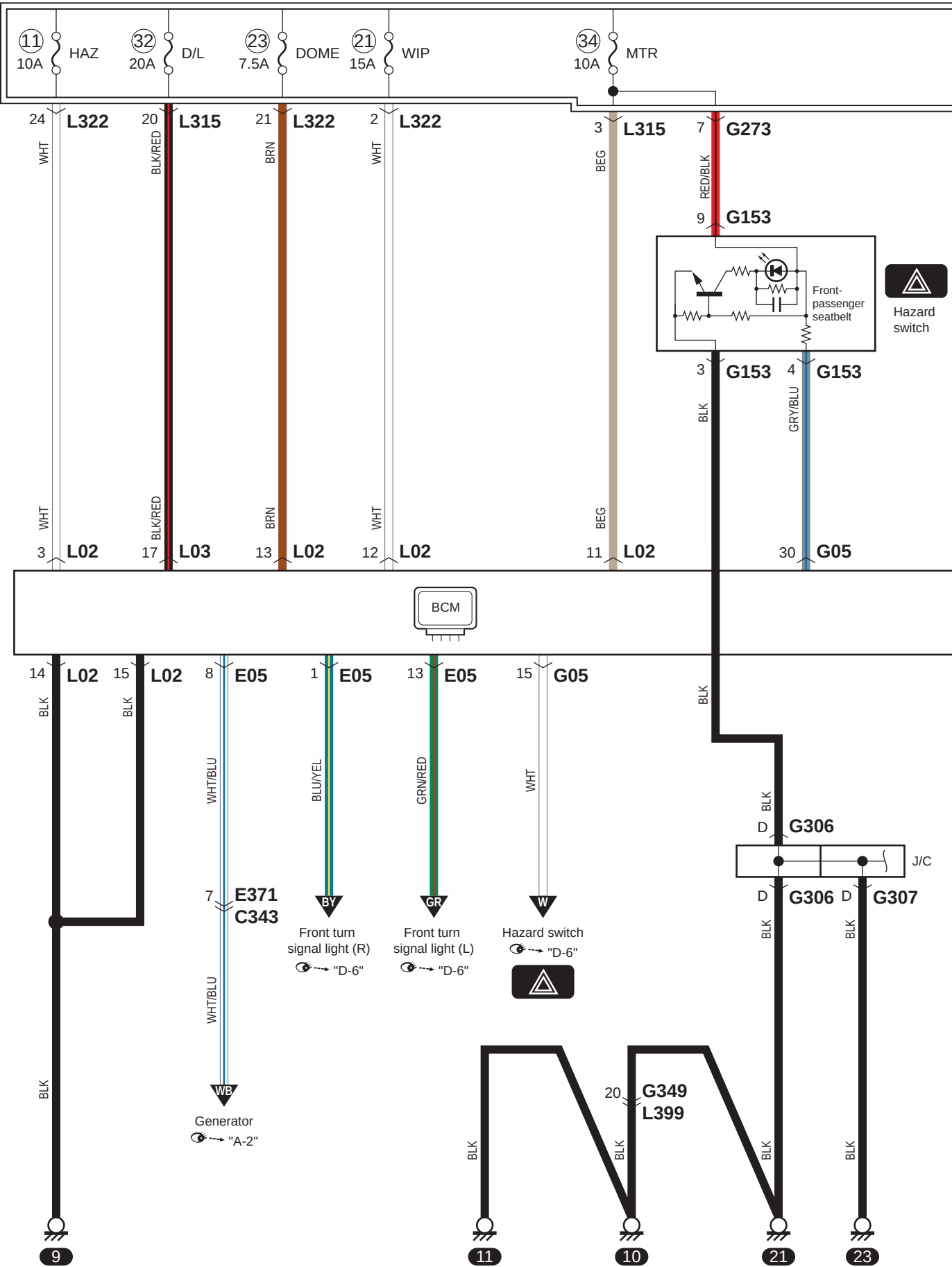
A-8-2 Diagrama del circuito del sistema de control de la carrocería (con sistema de arranque por pulsación del motor)
