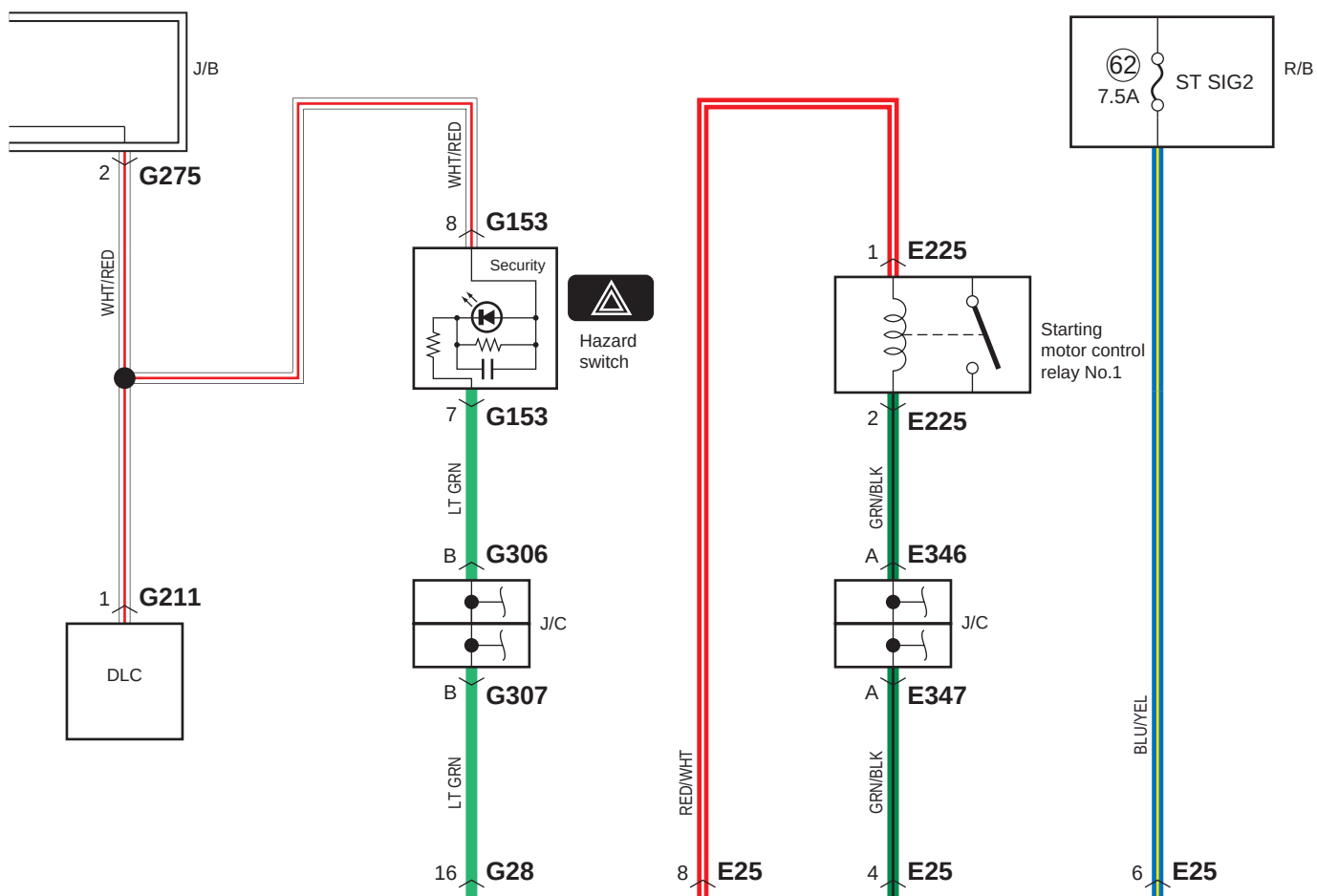
A-10 Diagrama del circuito del sistema de control de seguridad sin llaves (con sistema de arranque por pulsación del motor)
