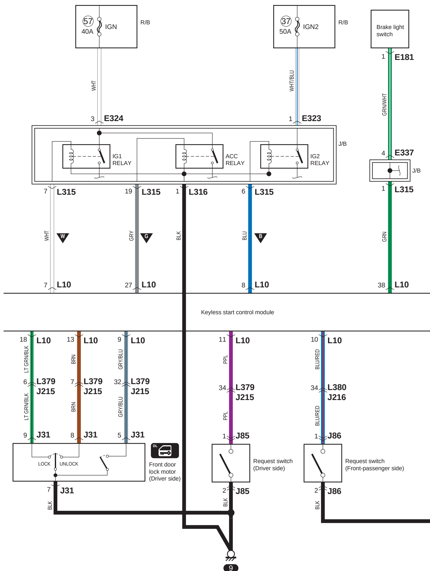
A-10 Diagrama del circuito del sistema de control de seguridad sin llaves (con sistema de arranque por pulsación del motor)
