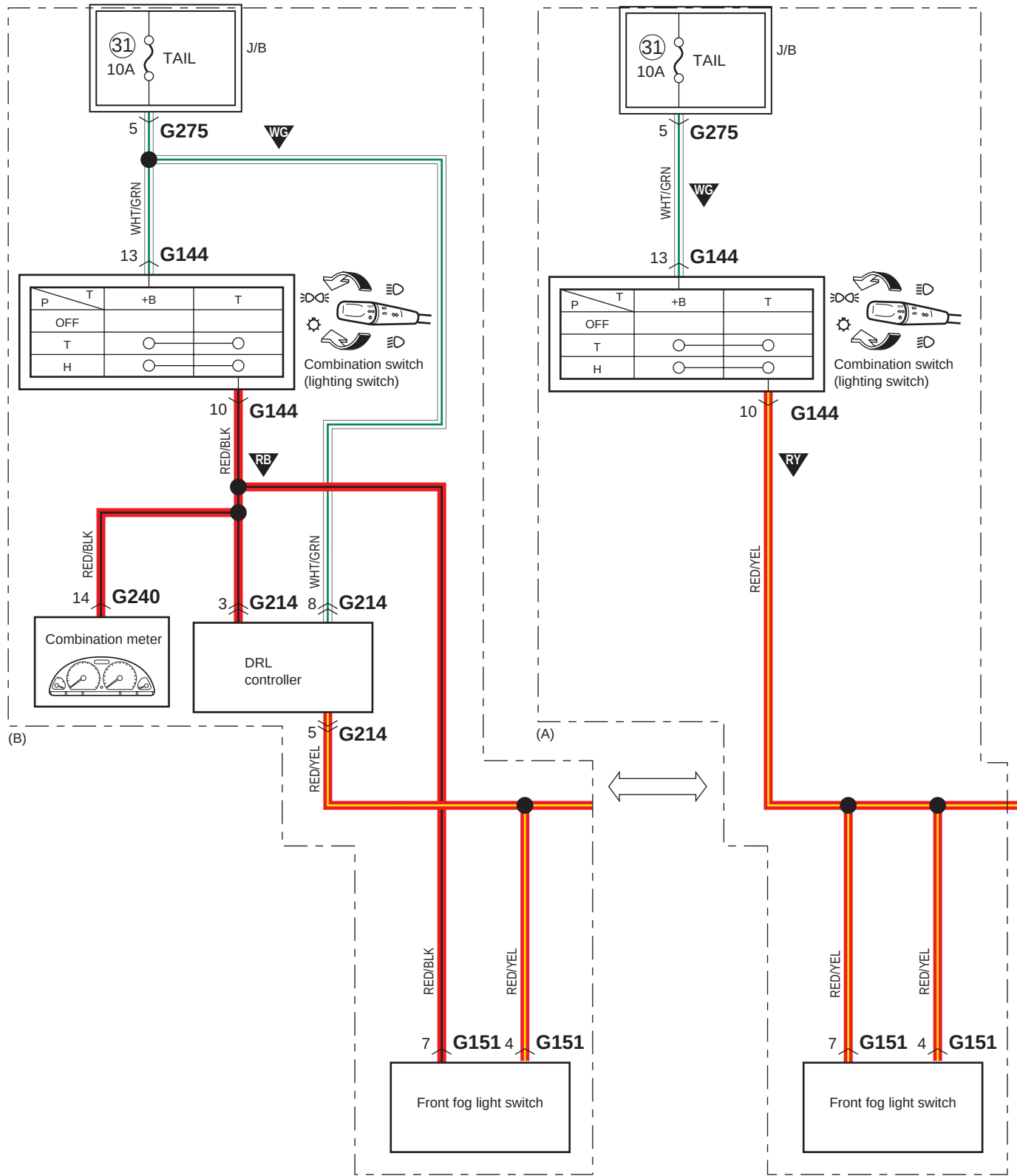
D-2-1 Diagrama del circuito del sistema de luz de la matrícula, de iluminación, de luces de posición y de luces traseras (sin sistema de arranque por pulsación del motor)
