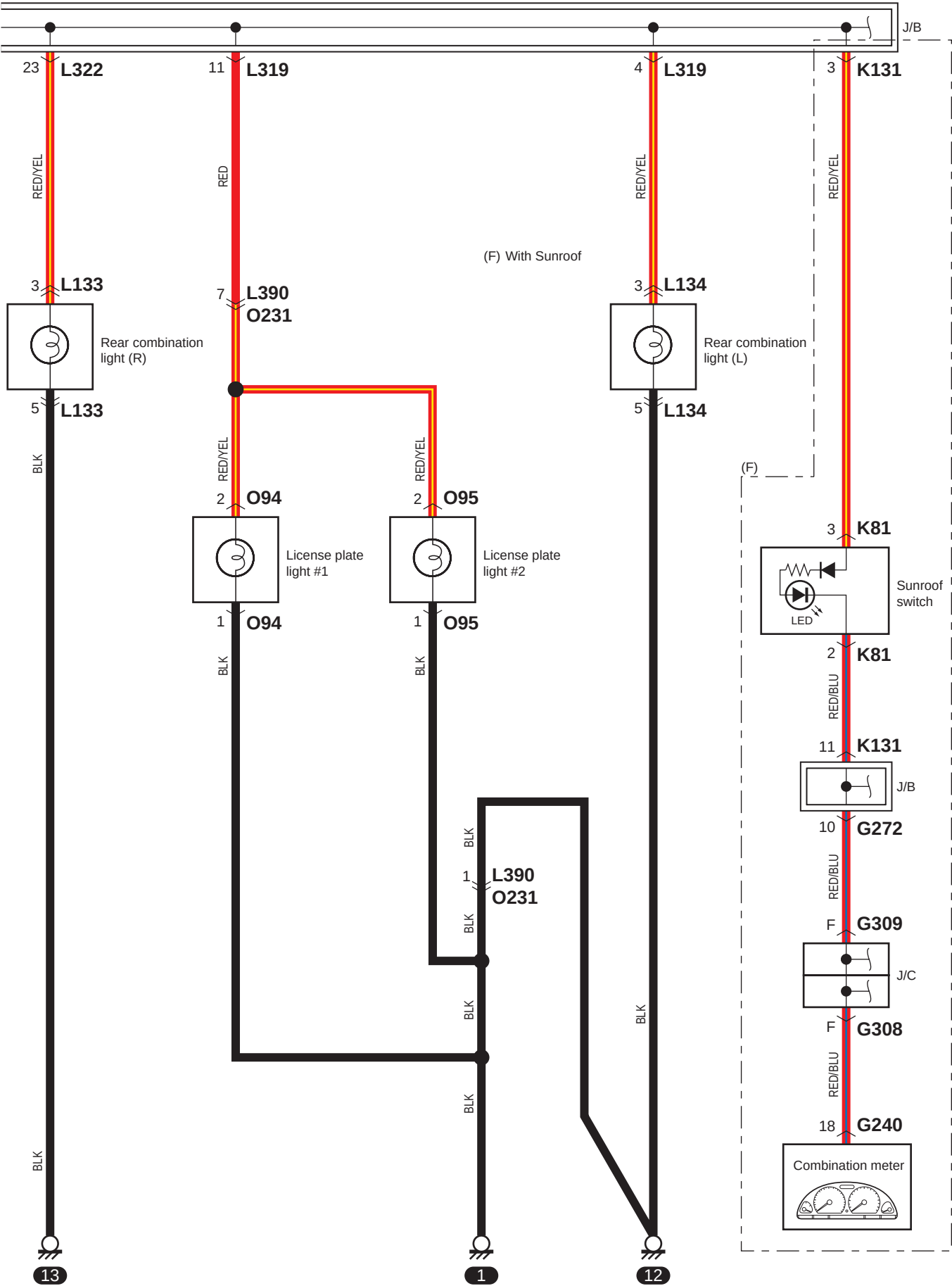
D-2-2 Diagrama del circuito del sistema de luz de la matrícula, de iluminación, de luces de posición y de luces traseras (con sistema de arranque por pulsación del motor)
