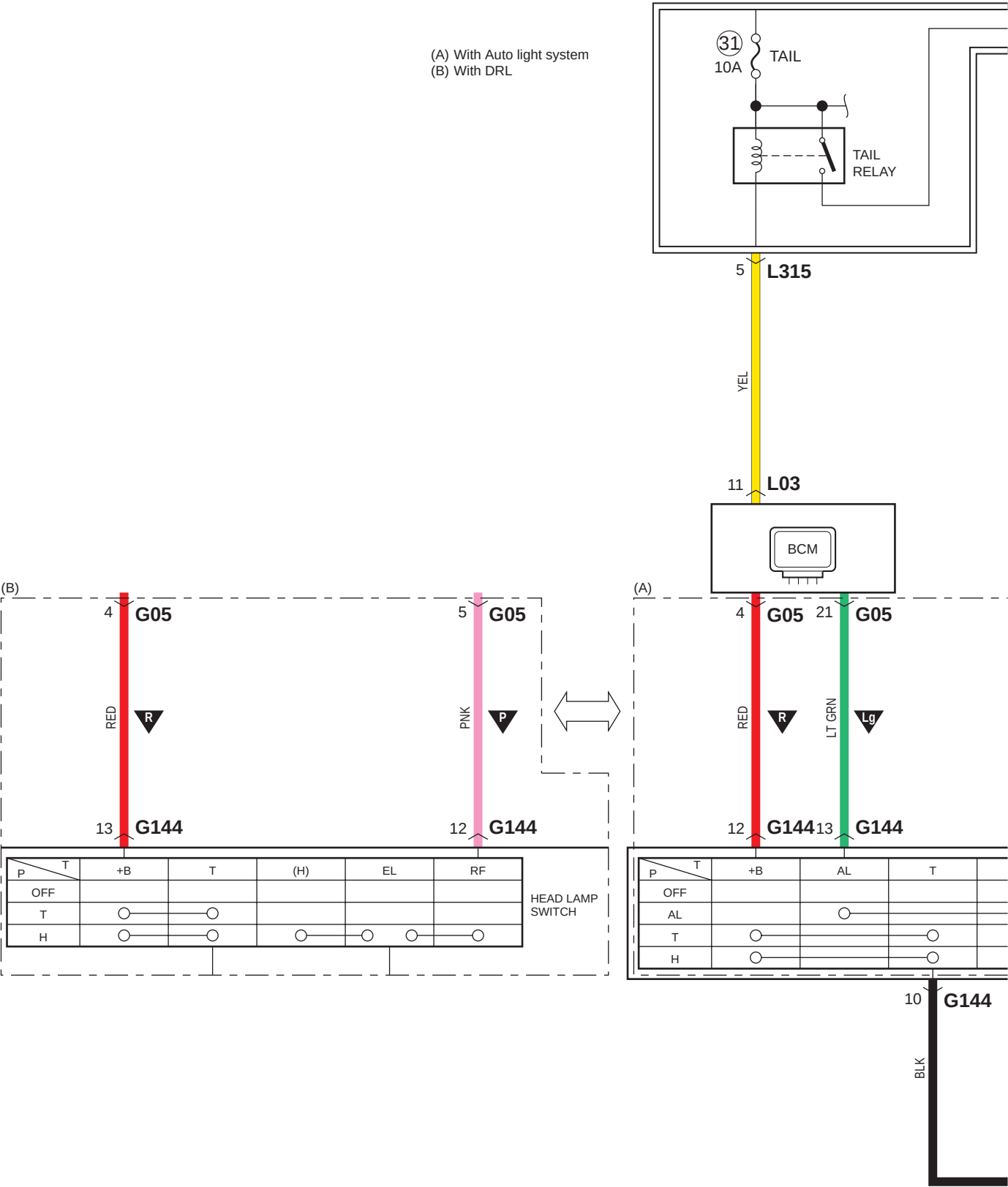
D-2-2 Diagrama del circuito del sistema de luz de la matrícula, de iluminación, de luces de posición y de luces traseras (con sistema de arranque por pulsación del motor)
