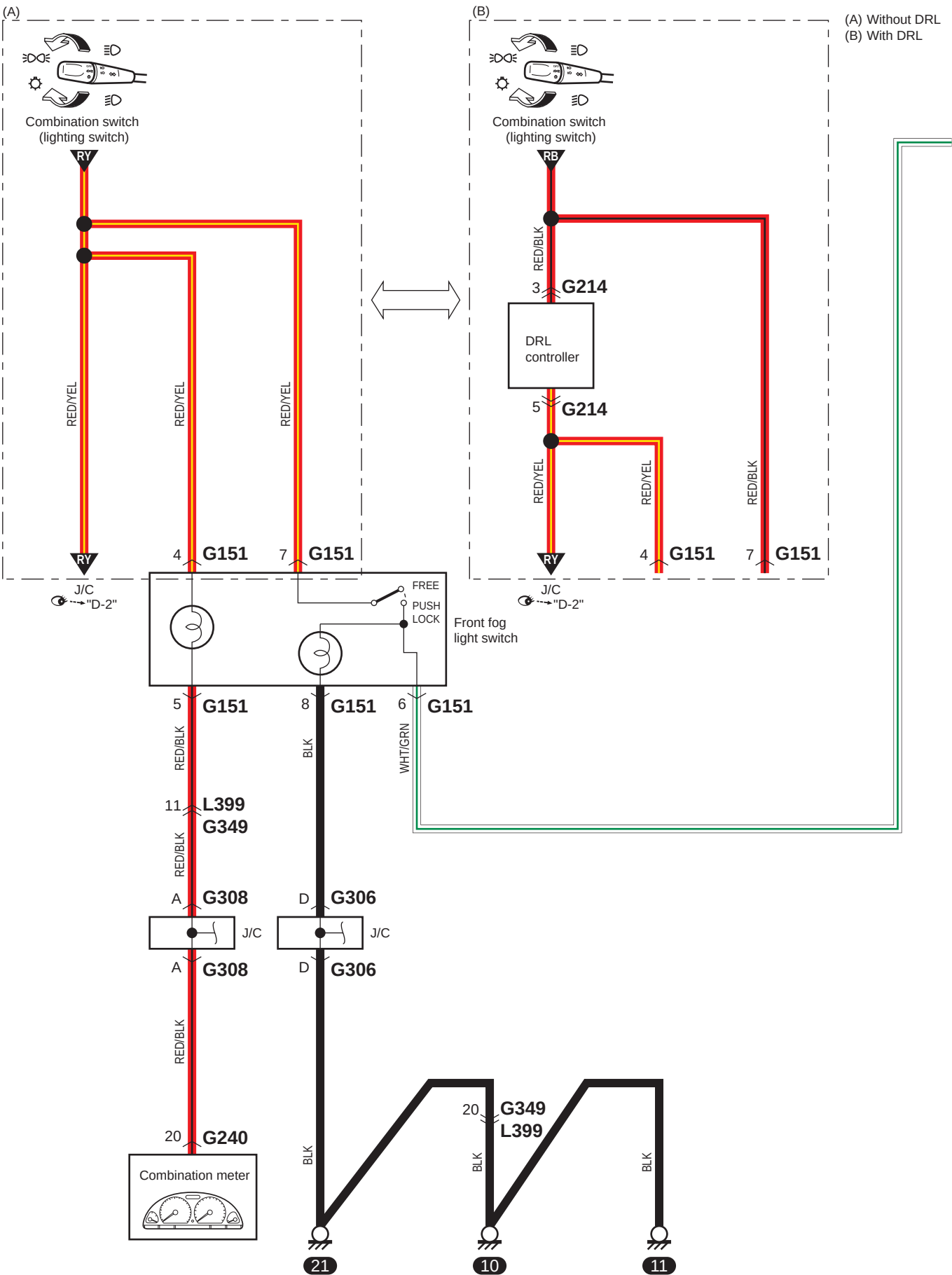
D-3-1 Diagrama del circuito del sistema de la luz antiniebla delantera (sin sistema de arranque por pulsación del motor)
