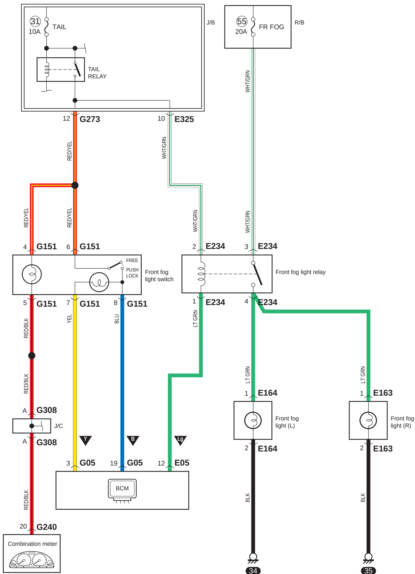
D-3-2 Diagrama del circuito del sistema de la luz antiniebla delantera (con sistema de arranque por pulsación del motor)
