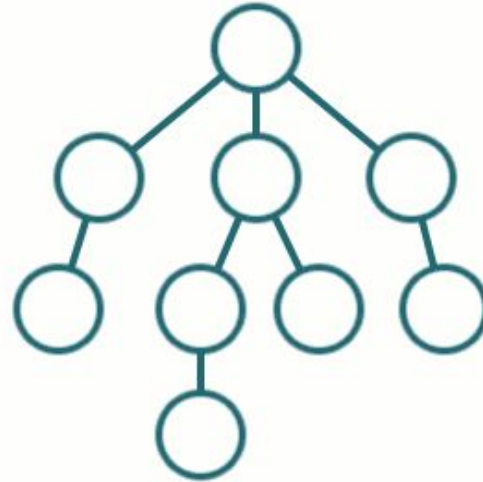
BFS
