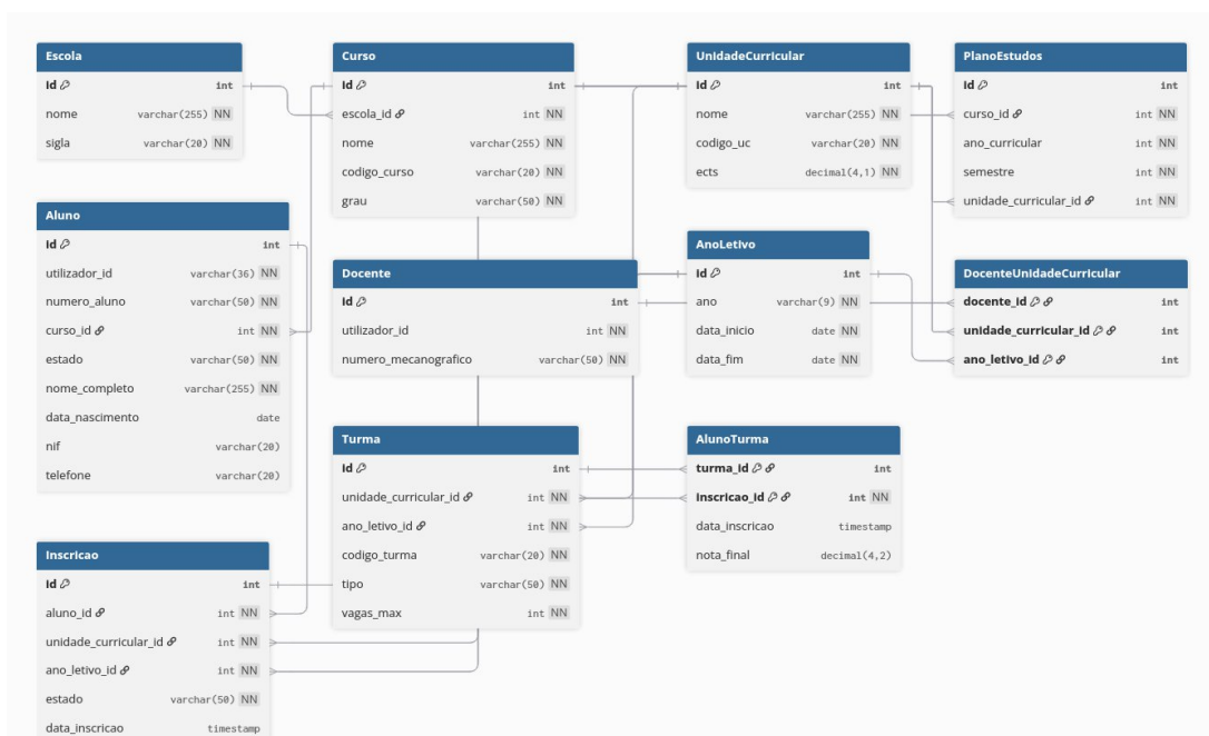
FIGURE 27 - BASE DE DADOS DO MICROSERVIÇO DE GESTÃO ACADÉMICA
