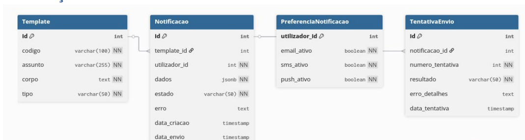
FIGURE 30 - BASE DE DADOS DO MICROSERVIÇO DE NOTIFICAÇÕES
