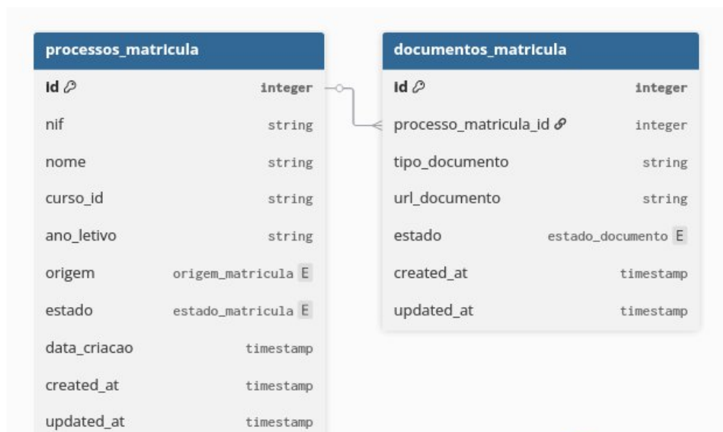
FIGURE 26 - BASE DE DADOS DO MICROSERVIÇO DE MATRÍCULAS
