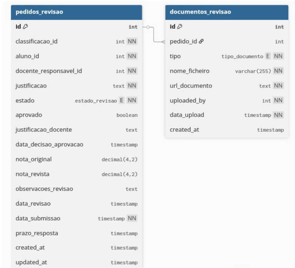
FIGURE 23 - BASE DE DADOS DO MICROSERVIÇO DE REVISÕES
