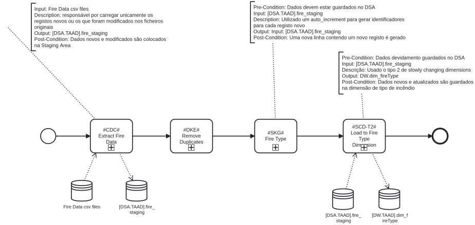
Figura 7. Diagrama BPMN nível padrão para a dimensão Tipo de Incêndio
