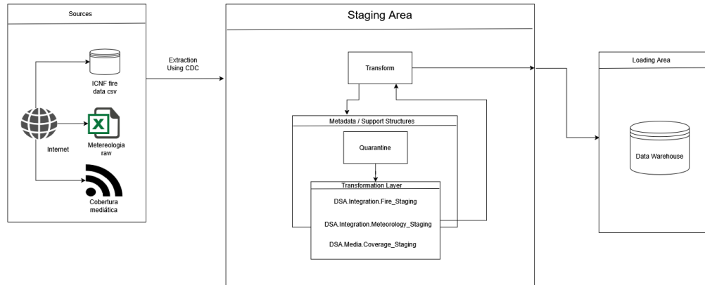
Figura 1. Arquitetura ELT (Estrutura da DSA)
