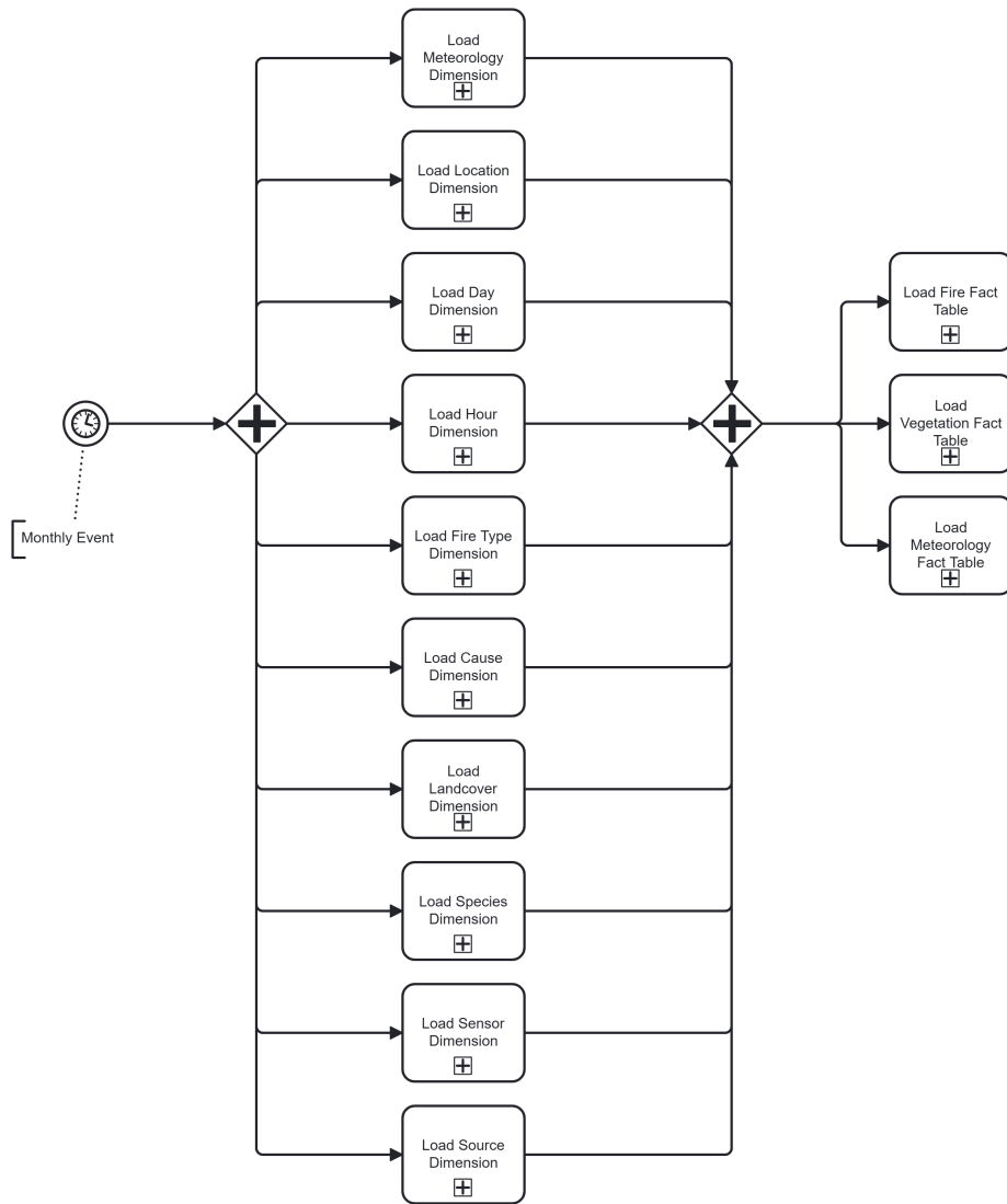
Figura 6. Diagrama BPMN ao nível do processo
