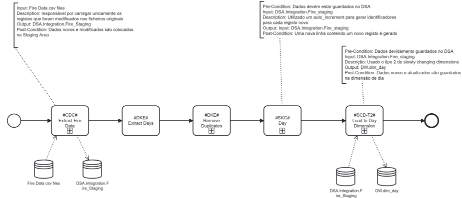
Figura 8. Diagrama BPMN nível padrão para dimensão dia
