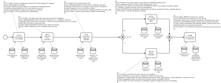
Figura 9. Diagrama BPMN nível padrão para tabela de factos de incêndio
