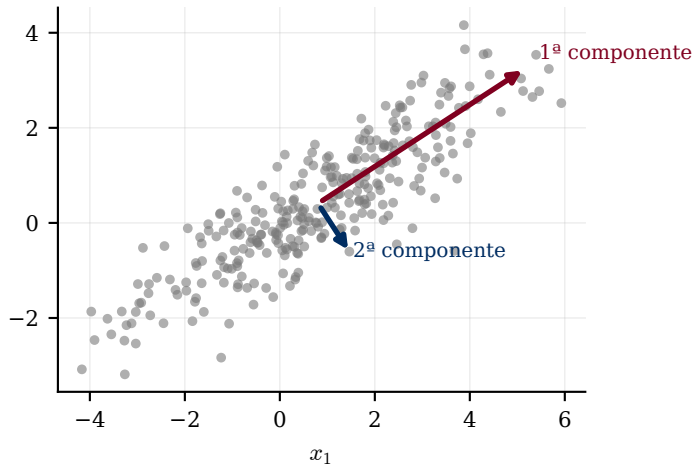
as direções de maior variância
