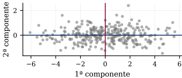
os mesmos dados, nas novas coordenadas
