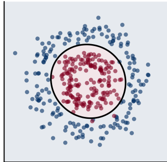
RBF, \gamma=0,5 acurácia (treino) = 0.994
