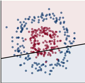
linear acurácia (treino) = 0.600
