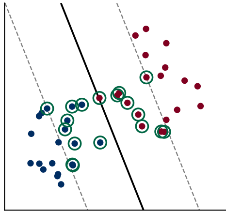
C=0.05 — 18 vetores de suporte margem = 2.80
