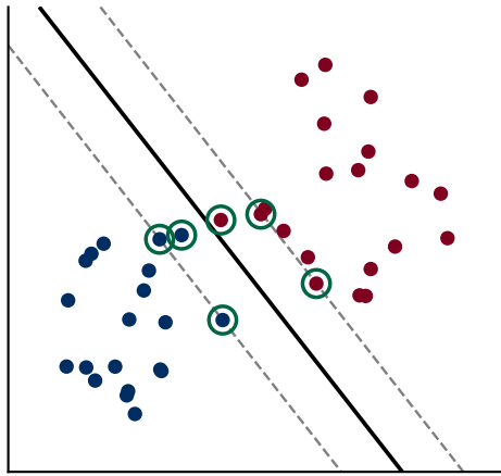
C=1 — 6 vetores de suporte margem = 1.16
