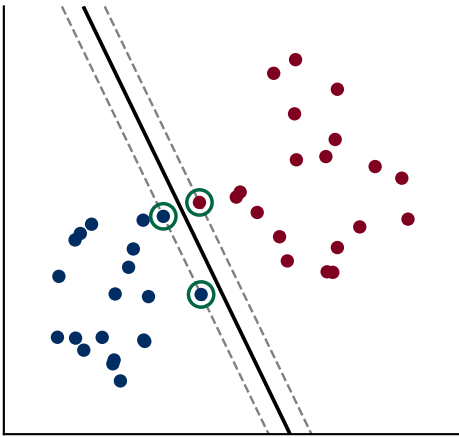
C=100 — 3 vetores de suporte margem = 0.50
