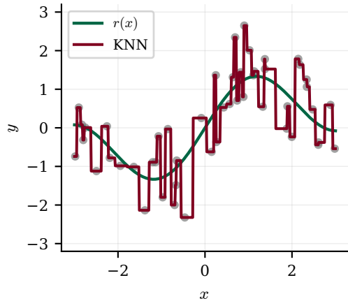
k=1 — superajuste
