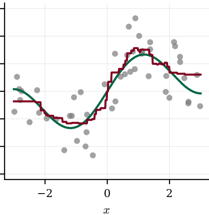
k=9 — equilíbrio
