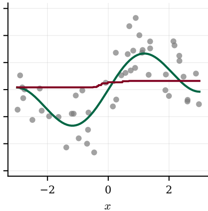
k=40 — subajuste
