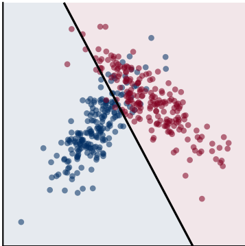
LDA (covariância comum)
