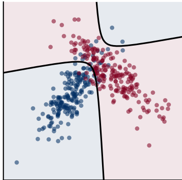
QDA (covariância por classe)
