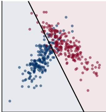
LDA (covariância comum)
