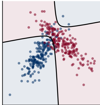
QDA (covariância por classe)
