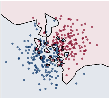
k = 1 treino 1.000 | teste 0.826
