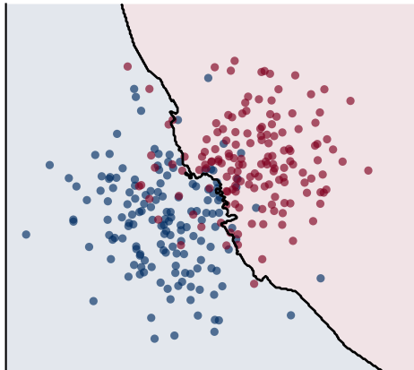
k = 15 treino 0.890 | teste 0.888
