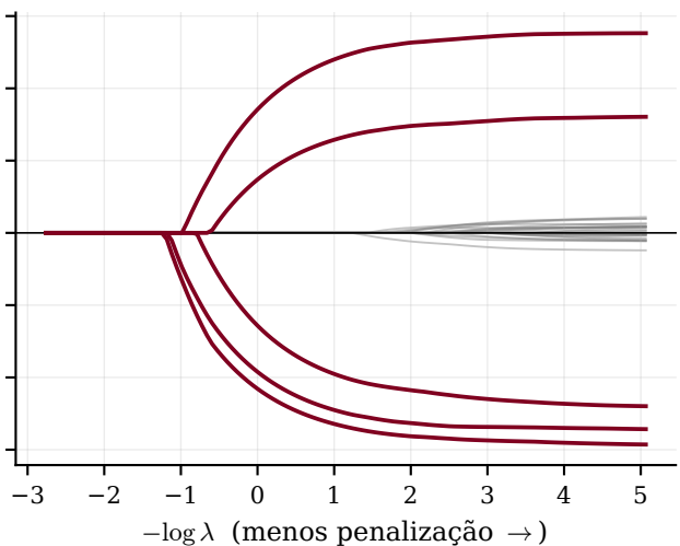
Lasso ( \ell_1 )
