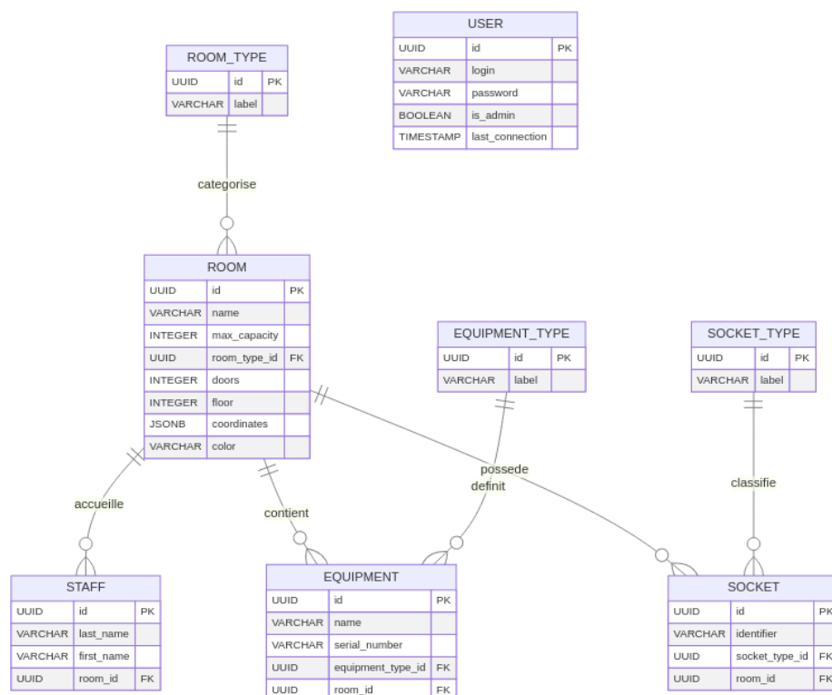
FIGURE 4.1 – Schéma relationnel de la base de données PostgreSQL
