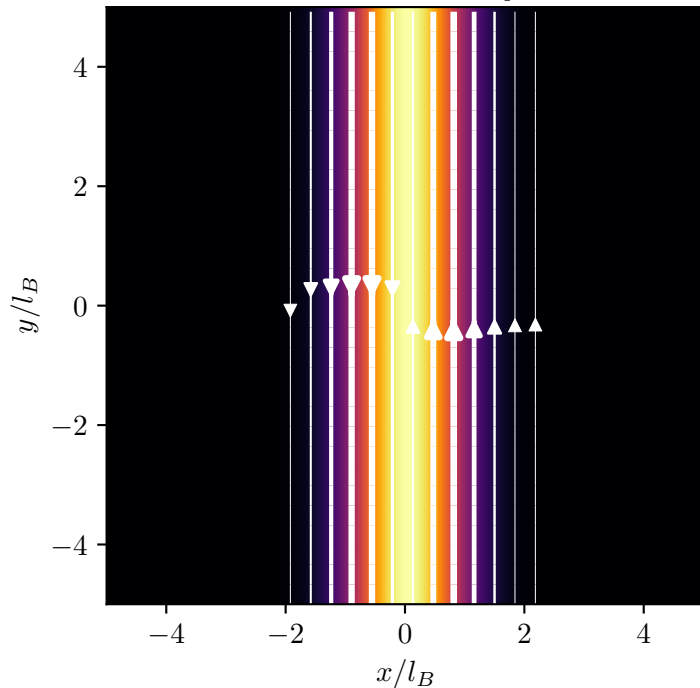
Spin Current \vec{J}_{spin}
