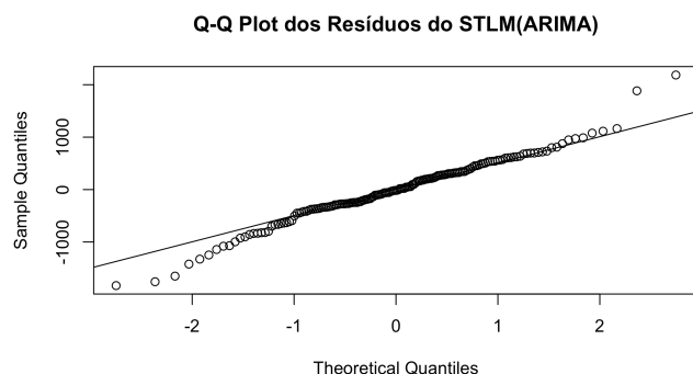
Figura 8: Gráfico QQ dos resíduos do modelo STLM.
