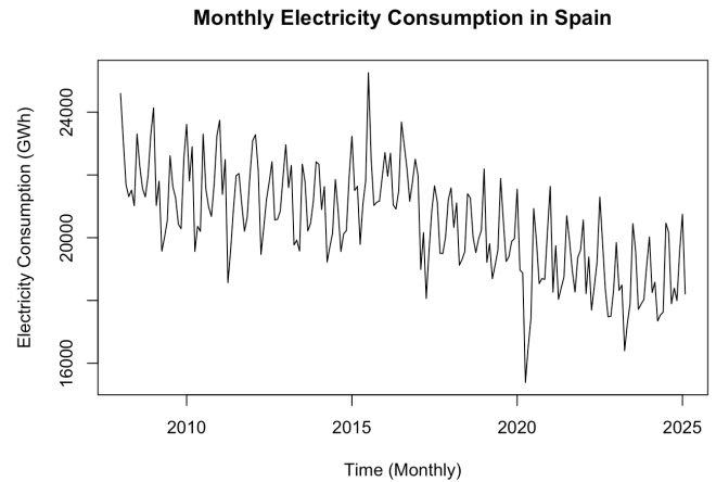
Figura 1: Série temporal univariada do consumo mensal de eletricidade em Espanha (2008–2025).
