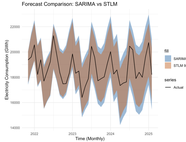
Figura 10: Intervalos de previsão a 95% para os modelos SARIMA e STLM.
