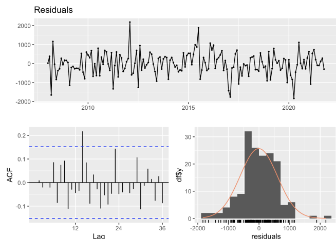
Figura 7: Análise dos resíduos do modelo STLM.
