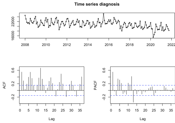
(a) Série original com respetiva ACF e PACF.
