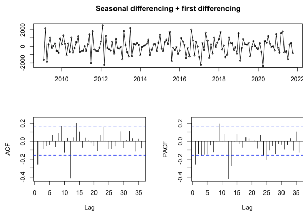
(b) Série diferenciada (ordem 1 e ordem 12) com respetiva ACF e PACF.
