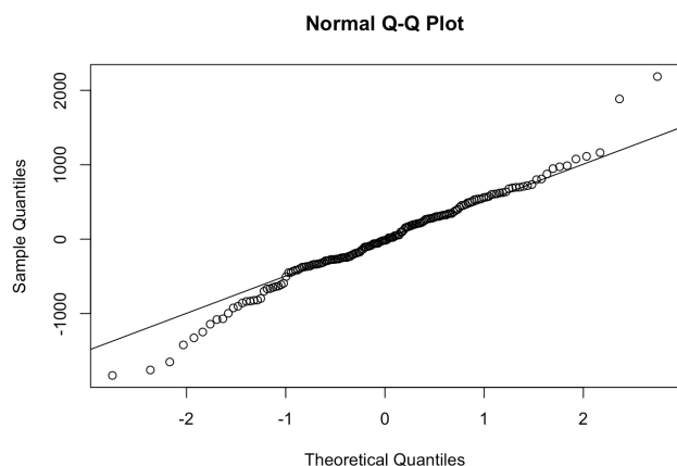
Figura 8: Gráfico QQ dos resíduos do modelo STLM.
