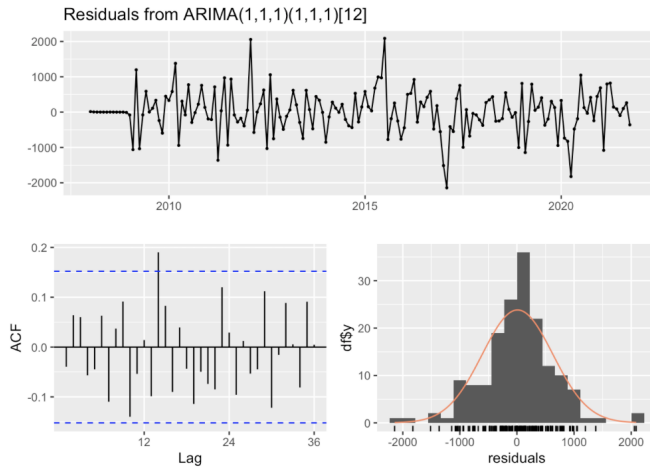
Figura 5: Análise dos resíduos do modelo SARIMA.
