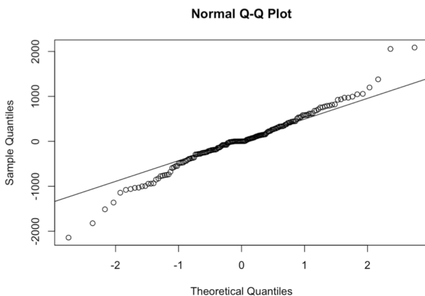
Figura 6: Gráfico QQ dos resíduos do modelo SARIMA.
