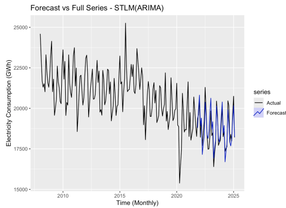
(b) Modelo STLM(ARIMA).
