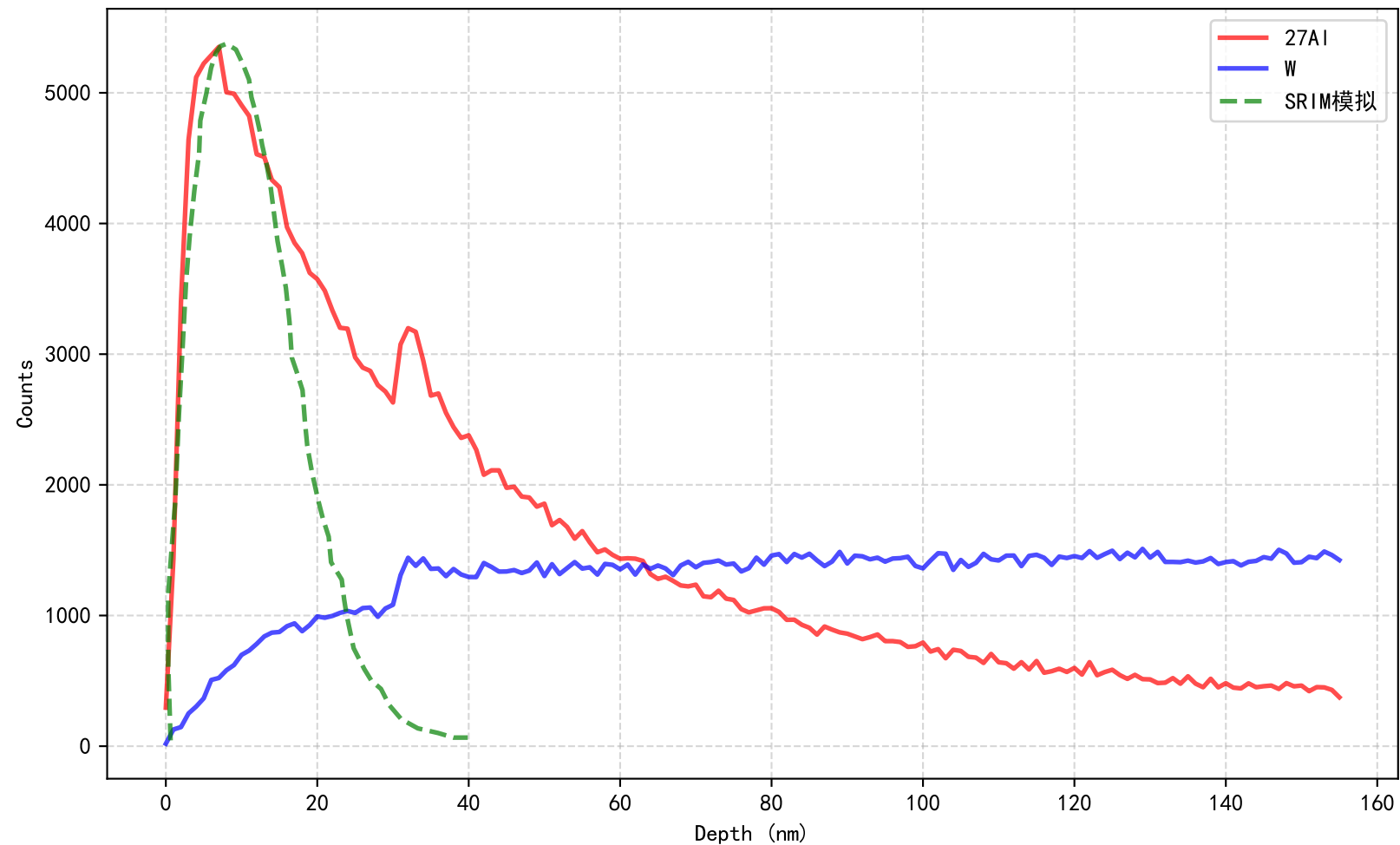
27Al和W的深度分布
