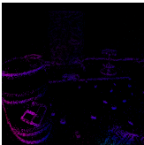
PLIF-EV-FlowNet
