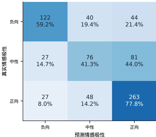
验证集情感极性混淆矩阵 ( 728条 )
