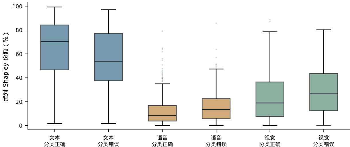
情感强度解释：分类正确与错误样本的模态作用
