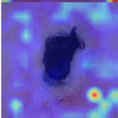
Grad-CAM (MPSA)
