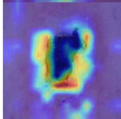
Grad-CAM (Ours)
