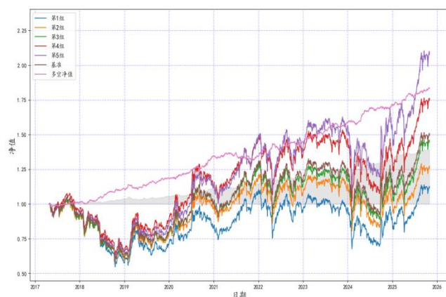
图 50：经营结构两因子净值--等权
