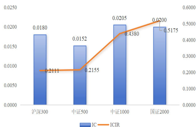
图 55：经营结构两因子各选股域 IC 和 ICIR 对比
