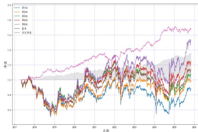
图 58：经营结构两因子中证 1000 选股净值
