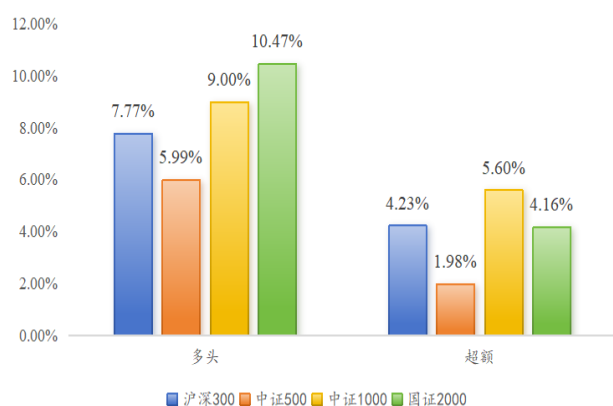
图 44：经营结构三因子各选股域多头和超额对比
