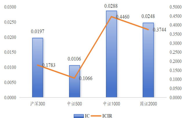
图 45：经营结构三因子各选股域 IC 和 ICIR 对比
