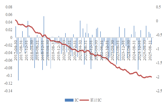
图 28：主要客户占比因子 Rank IC
