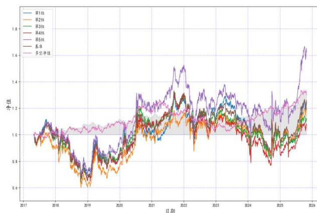
图 9：外币资金占比因子中证 500 选股净值
