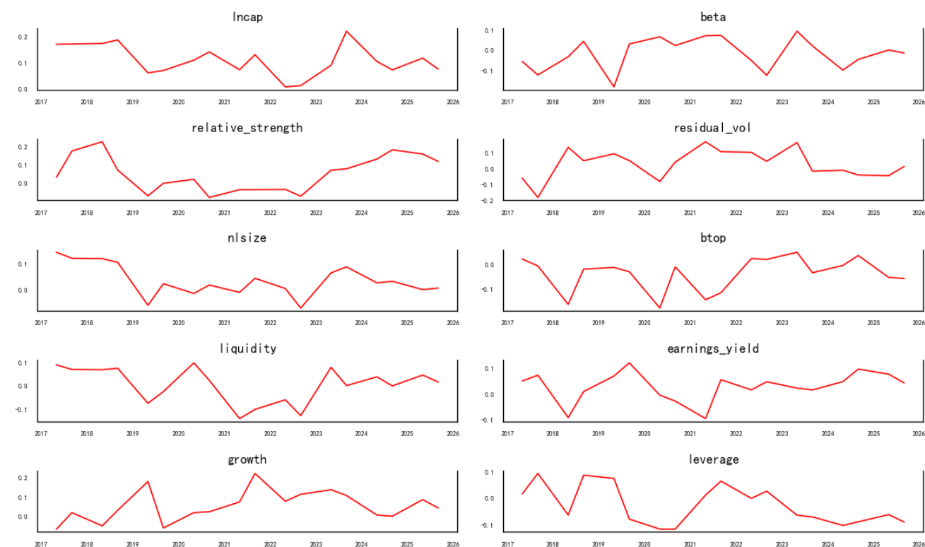
图 18：境外收入占比因子多头组与 Barra 风格因子秩相关性序列
