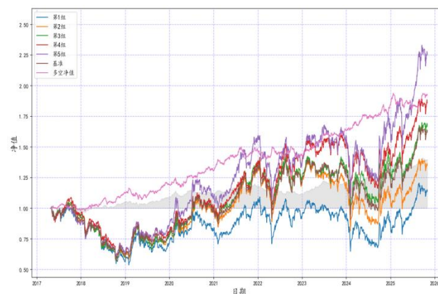
图 49：经营结构三因子国证 2000 选股净值
