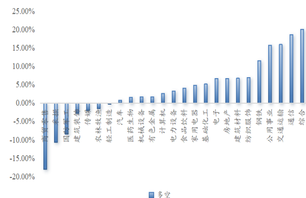
图 25：境外收入占比因子分行业多空年化
