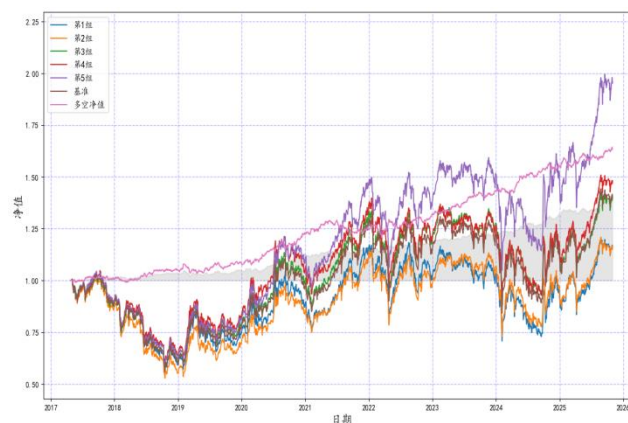
图 59：经营结构两因子国证 2000 选股净值
