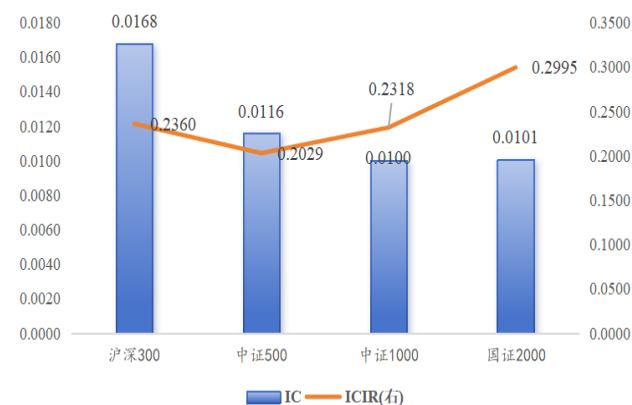
图 7：外币资金占比因子各选股域 IC 和 ICIR 对比
