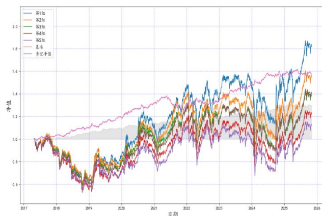
图 37：主要客户占比因子国证 2000 选股净值
