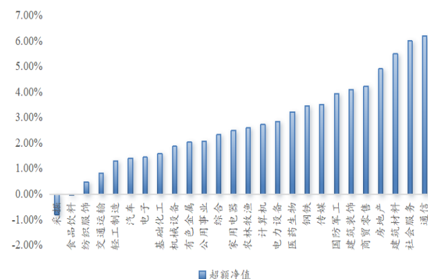
图 13：外币资金占比因子分行业超额年化
