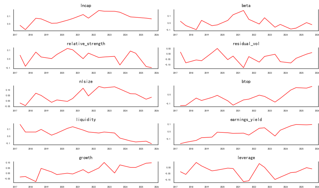
图 31：主要客户占比因子多头组与 Barra 风格因子秩相关性序列
