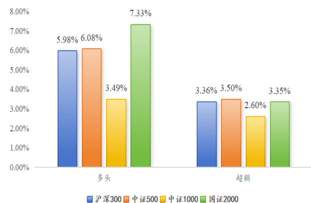
图 6：外币资金占比因子各选股域多头和超额对比
