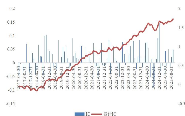
图 15：境外收入占比因子 Rank IC
