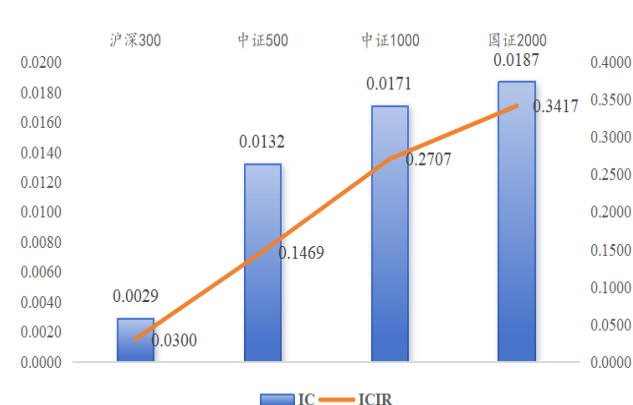
图 20：境外收入占比因子各选股域 IC 和 ICIR 对比
