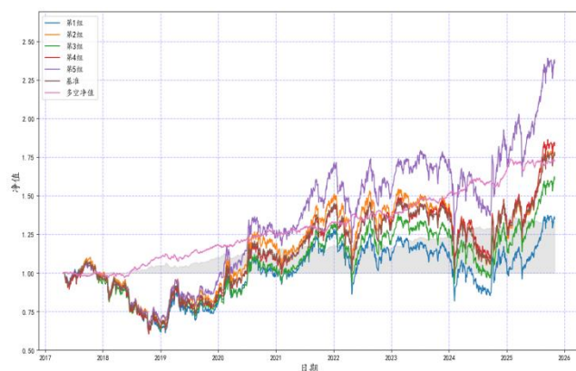
图 14：境外收入占比因子净值--等权
