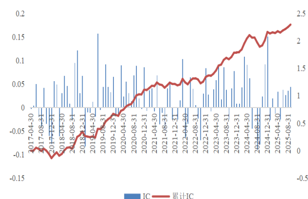
图 41：经营结构三因子 Rank IC
