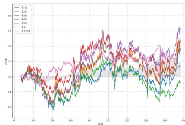
图 47：经营结构三因子中证 500 选股净值
