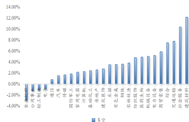
图 38：主要客户占比因子分行业多空年化
