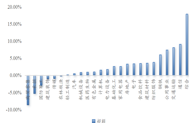
图 26：境外收入占比因子分行业超额年化
