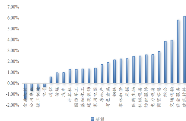
图 39：主要客户占比因子分行业超额年化
