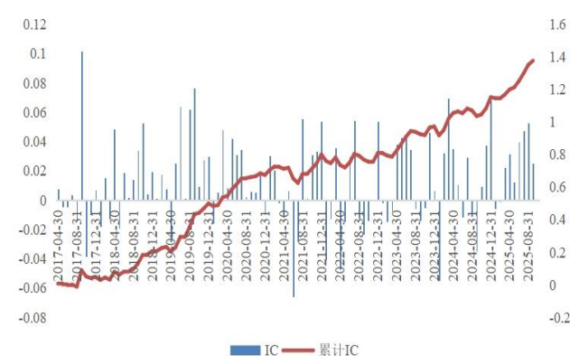
图 2: 外币资金占比因子 Rank IC
