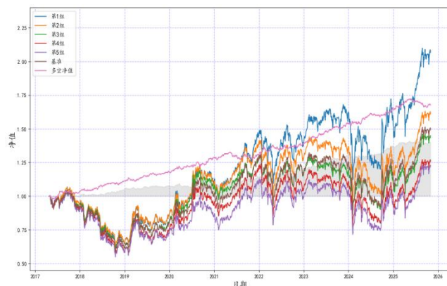
图 27：主要客户占比因子净值--等权
