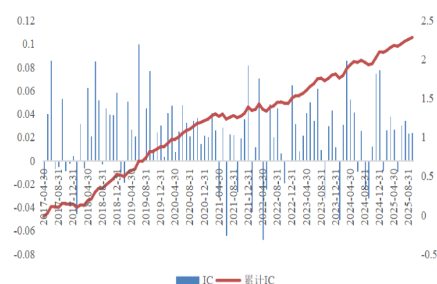
图 51：经营结构两因子 Rank IC
