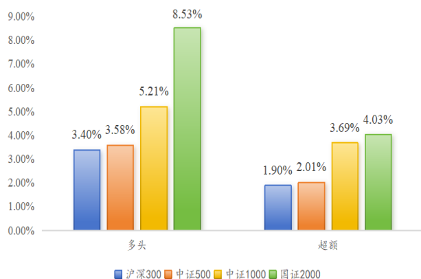
图 54：经营结构两因子各选股域多头和超额对比
