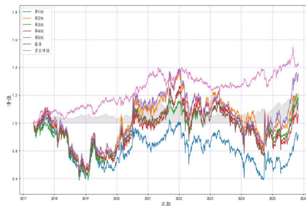
图 57：经营结构两因子中证 500 选股净值
