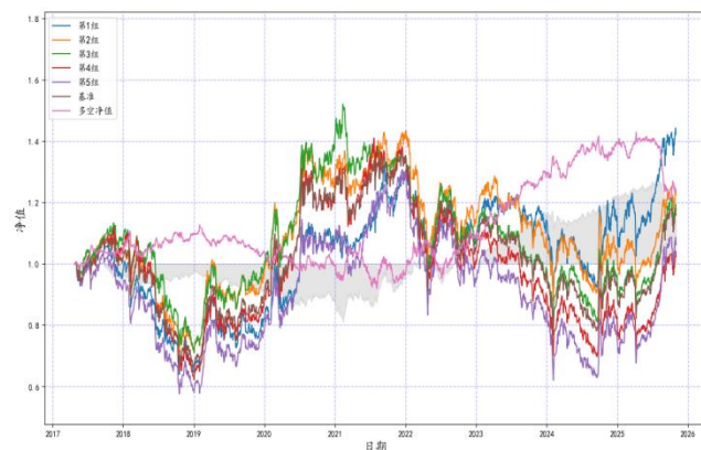
图 29：主要客户占比因子净值--市值加权
