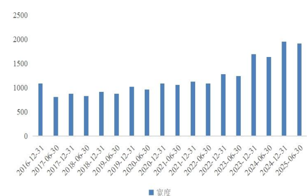
图 17：境外收入占比因子宽度
