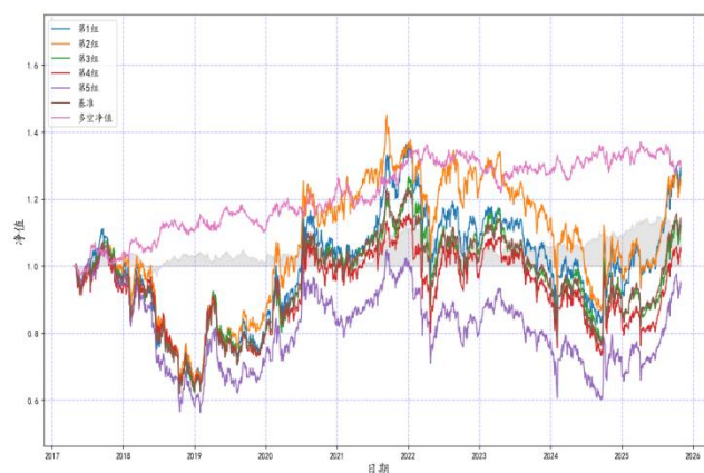
图 35：主要客户占比因子中证 500 选股净值
