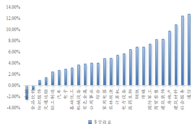
图 12：外币资金占比因子分行业多空年化
