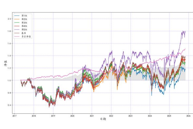
图 11：外币资金占比因子国证 2000 选股净值
