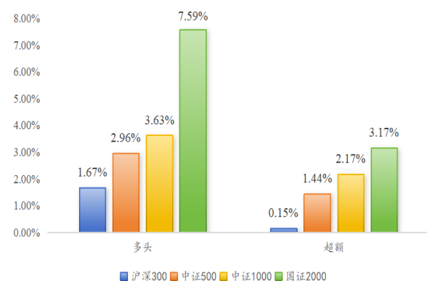
图 32：主要客户占比因子各选股域多头和超额对比
