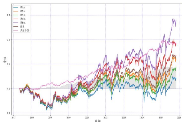
图 24：境外收入占比因子国证 2000 选股净值
