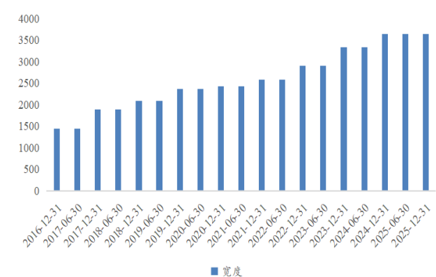
图 30：主要客户占比因子宽度
