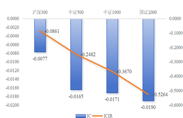
图 33：主要客户占比因子各选股域 IC 和 ICIR 对比
