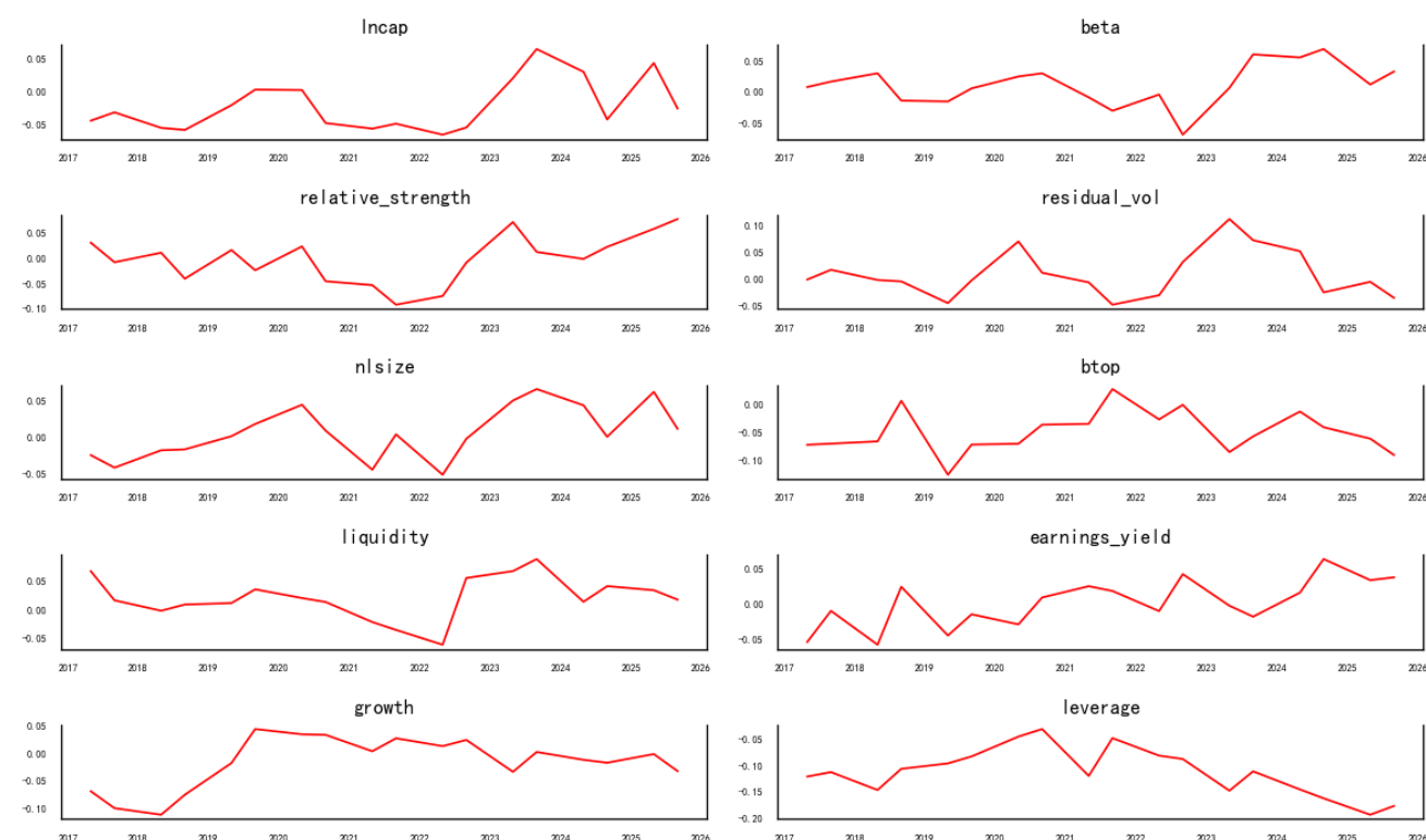
图 5：外币资金占比因子多头组与 Barra 风格因子秩相关性序列
