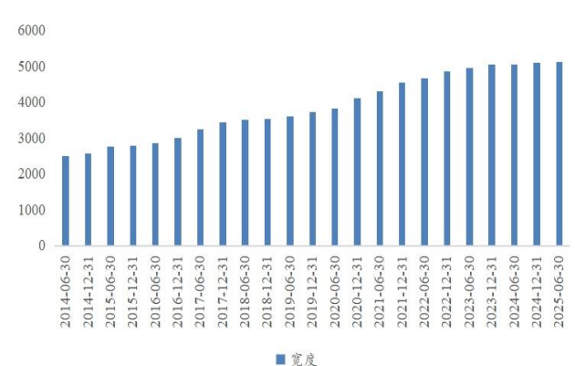
图 4：外币资金占比因子宽度
