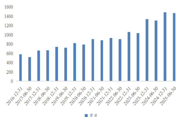
图 43：经营结构三因子宽度
