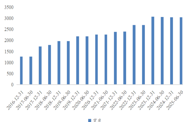
图 53：经营结构两因子宽度
