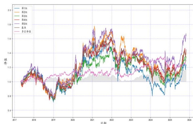
图 16：境外收入占比因子净值--市值加权
