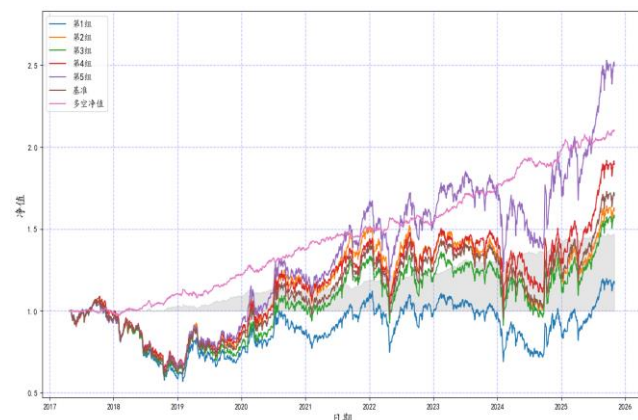
图 40：经营结构三因子净值--等权
