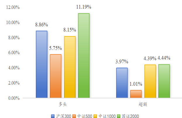
图 19：境外收入占比因子各选股域多头和超额对比
