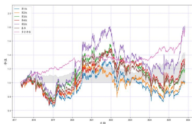
图 3：外币资金占比因子净值--市值加权
