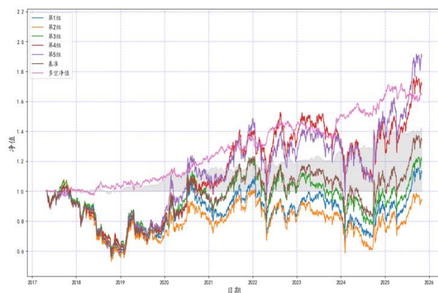
图 23：境外收入占比因子中证 1000 选股净值
