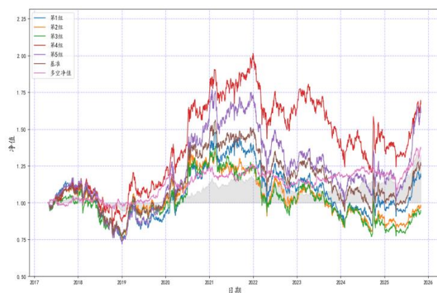
图 8：外币资金占比因子沪深 300 选股净值
