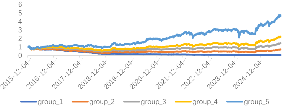
alpha158策略
