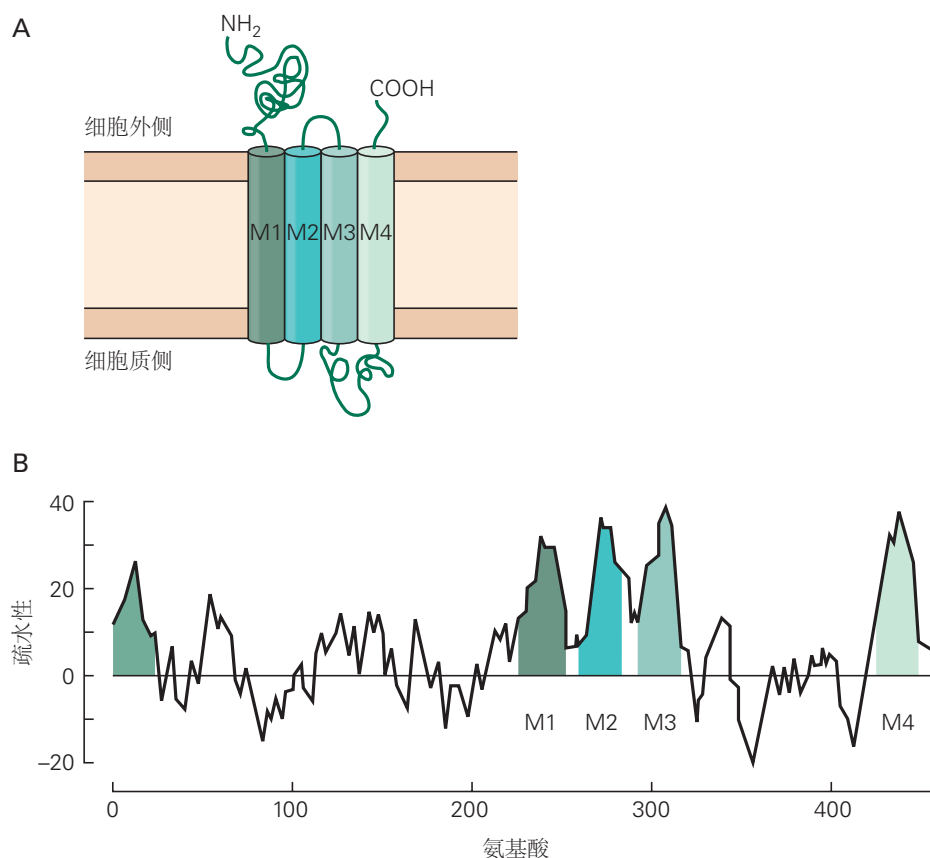
图 8.3.2: 跨膜蛋白的二级结构。A. 骨骼肌中存在的烟碱乙酰胆碱受体通道亚基的二级结构。每个圆柱体 (M1–M4) 代表一个假定的跨膜 \alpha -螺旋，由大约 20 个疏水氨基酸残基组成。膜片段由亲水性残基的细胞质或细胞外片段 (环) 连接。蛋白质的氨基末端 ( \text{NH}_2 ) 和羧基末端 ( \text{COOH} ) 位于膜的细胞外侧。B. 离子通道蛋白的跨膜区域可以使用疏水性图来识别。从克隆的受体亚基基因的核苷酸序列推断出烟碱型乙酰胆碱受体 \alpha -亚基的氨基酸序列。然后绘制亚基整个氨基酸序列的疏水性移动平均值。图中的每个点代表 19 个氨基酸序列的平均疏水指数，对应于序列的中点。4 个疏水区域 (M1–M4) 对应于跨膜片段。图中最左边的疏水区域是信号序列，在蛋白质合成过程中，它将蛋白质的亲水氨基末端定位在细胞的外表面。信号序列从成熟蛋白上切下 [45] 。
