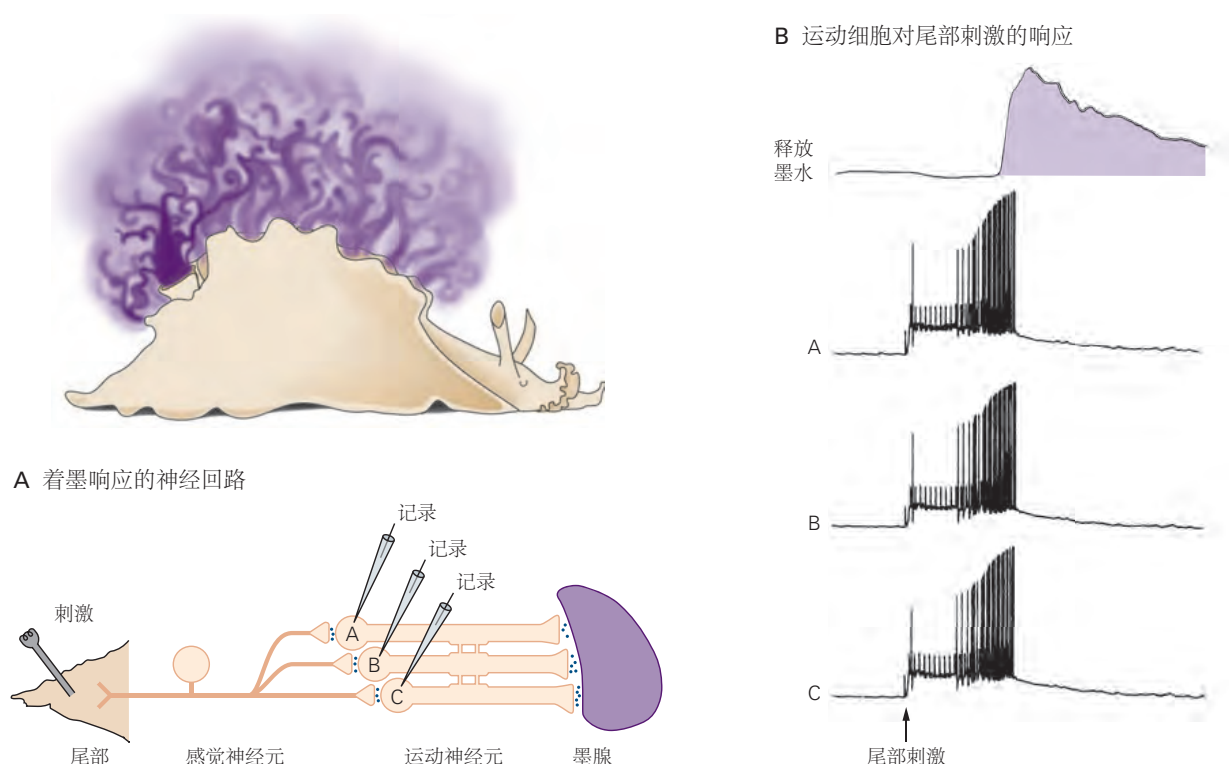
图 11.2.6: 一起放电的电耦合运动神经元可以产生同步行为 [65] 。A. 在海螺海兔中，来自尾部神经节的感觉神经元与支配墨腺的 3 个运动神经元形成突触。运动神经元通过电突触相互连接。B. 应用于尾部的一系列刺激会在所有 3 个运动神经元中产生同步放电，从而导致墨水释放。
