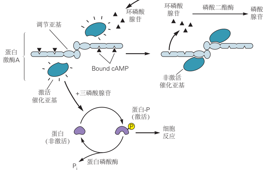
图 14.1.1: G 蛋白偶联受体的激活会刺激环磷酸腺苷的产生和蛋白激酶 A [7] 。A. 递质与某些受体的结合会激活刺激性 G 蛋白 ( G_s )，包括 \alpha_s -亚基、 \beta -亚基和 \gamma -亚基。当被激活时， \alpha_s 亚基将其结合的二磷酸鸟苷交换为三磷酸鸟苷，导致 \alpha_s 从 \beta\gamma 复合物中解离。接下来， \alpha_s 与腺苷酸环化酶的胞内结构域结合，从而刺激该酶从三磷酸腺苷产生环磷酸腺苷。三磷酸鸟苷水解为二磷酸鸟苷和无机磷酸盐 ( P_i ) 导致 \alpha_s 从环化酶解离并与 \beta\gamma 复合物重新结合。然后环化酶停止产生第二信使。当递质与受体分离时，G 蛋白的 3 个亚基重新结合， \alpha 亚基上的鸟嘌呤核苷酸结合位点被二磷酸鸟苷占据。B. 4 个环磷酸腺苷分子与蛋白激酶 A 的 2 个调节亚基结合，释放 2 个催化亚基，然后自由磷酸化某些丝氨酸或苏氨酸残基上的特定底物蛋白，从而调节蛋白质功能以产生给定的细胞回复。有 2 种酶调节该通路。磷酸二酯酶将环磷酸腺苷转化为腺苷一磷酸 (无活性)，蛋白磷酸酶从底物蛋白中去除磷酸基团 (P)，释放无机磷酸盐 P_i 。当磷酸酶被蛋白激酶 A 磷酸化时，其活性又会被蛋白抑制剂 1 (未显示) 降低。
