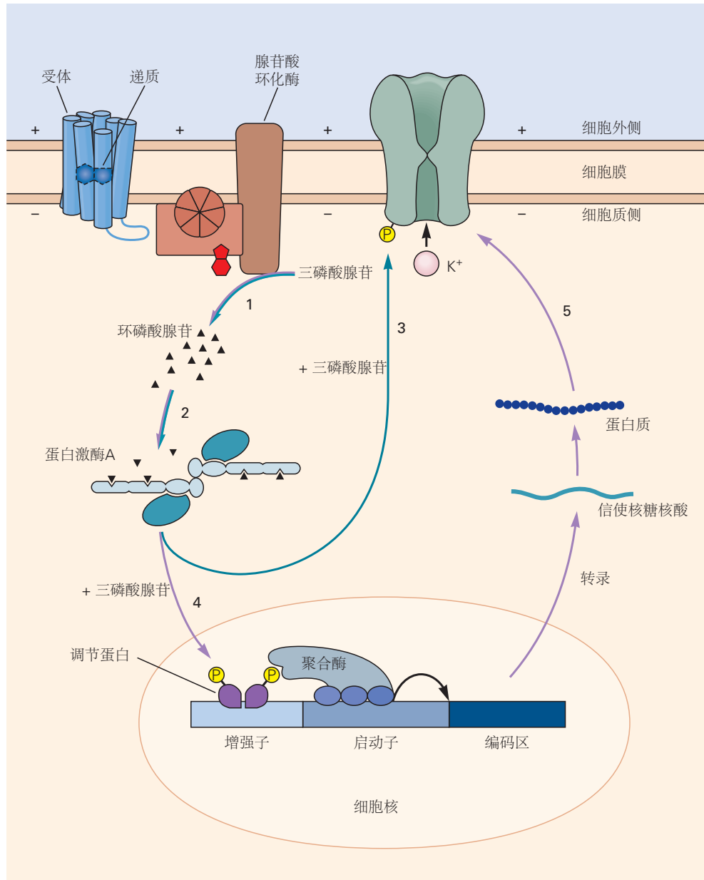
图 14.6.1: 单一的神经递质可以对离子通道产生短期或长期的影响。在此示例中，短时间接触递质会激活环磷酸腺苷第二信使系统 (1)，进而激活蛋白激酶 A (2)。激酶磷酸化 K^+ 通道；这会导致持续几分钟的突触电位并改变神经元的兴奋性 (3)。随着受体的持续激活，激酶转移到细胞核，在那里磷酸化一种或多种开启基因表达的转录因子 (4)。作为新蛋白质合成的结果，突触动作被延长，即通道的关闭和神经元兴奋性的变化持续数天或更长时间 (5)。
