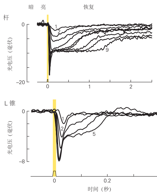
图 22.2.1: 光转导。 A. 视杆细胞对光有响应。外段视盘中的视紫红质分子吸收光子, 导致细胞质膜中环磷酸鸟苷门控通道关闭。这种通道关闭使膜超极化并降低神经递质谷氨酸的释放速率 [7] 。 B. 1. 光转导中的分子过程。环磷酸鸟苷由鸟苷酸环化酶从三磷酸鸟苷产生并被磷酸二酯酶水解。在黑暗中, 磷酸二酯酶活性低, 环磷酸鸟苷浓度高, 环磷酸鸟苷门控通道开放, 允许 \text{Na}^+ 和 \text{Ca}^{2+} 流入。在光线下, 视紫红质通过吸收光子而被激发, 然后激活转导蛋白, 转导蛋白进而激活磷酸二酯酶; 环磷酸鸟苷水平下降, 膜通道关闭, 更少的 \text{Na}^+ 和 \text{Ca}^{2+} 进入细胞。转导酶均位于内膜圆盘中, 可溶性配体环磷酸鸟苷作为细胞质膜的信使。 2. \text{Ca}^{2+} 在光转导响应级联中具有负反馈作用。光对网络的刺激导致环磷酸鸟苷门控通道的关闭。这导致细胞内 \text{Ca}^{2+} 浓度下降。因为 \text{Ca}^{2+} 调节至少 3 个级联组分的功能 (视紫红质、鸟苷酸环化酶和环磷酸鸟苷门控通道) \text{Ca}^{2+} 的下降抵消了光引起的激发。 C. 灵长类视杆细胞和视锥细胞对强度增加的短暂闪光的电压响应。迹线上的数字越高表示光照强度越大 (并非所有迹线都已标记)。对于昏暗的闪光, 响应幅度随强度线性增加。在高强度下, 受体饱和并在闪光后的一段时间内稳定地保持超极化; 这会导致我们在明亮的闪光后看到的残像。请注意, 对于更亮的闪光, 响应峰值更早, 并且视锥细胞的响应速度比视杆细胞快 [196] 。
