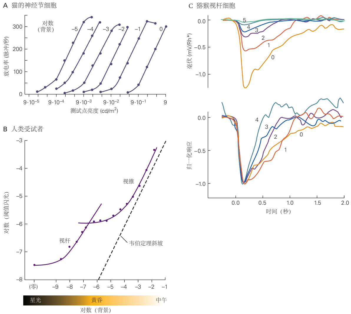
图 22.5.2: 光照适应。 A. 猫视网膜神经节细胞的感受野在稳定的背景强度下均匀照明，并在感受野中心短暂闪烁一个测试点。测量闪光后的峰值激活率并根据闪光强度的对数绘制。每条曲线对应不同的背景强度，从左到右增加 10 倍 [199] 。B. 一个小的测试点在稳定照明的背景上短暂闪光，闪光强度逐渐增加到人类受试者刚好可以检测到的程度。在不同的背景强度下重复该过程。这里，阈值闪光强度根据背景强度绘制。该曲线有 2 个分支，由一个明显的扭结相连：它们对应于视杆视觉和视锥视觉的状态。当阈值强度与背景强度成正比时，韦伯定律的斜率表示理想化 [200] 。C. 上图显示了猕猴视杆细胞对不同背景强度下出现闪光的响应。细胞的单光子响应根据记录的膜电位除以闪光激活的视紫红质的数量计算得出。单光子响应的增益随着背景强度的增加而显著降低。背景强度（以光子/平方微米/秒为单位）对于迹线 0 为 0，对于迹线 1 为 3.1，对于迹线 2 为 12，对于迹线 3 为 41，对于迹线 4 为 84，对于迹线 5 为 162。在底部图中，相同数据（最小响应除外）被归一化为相同的振幅，表明单光子响应的时间进程在高强度下加速 [201] 。
