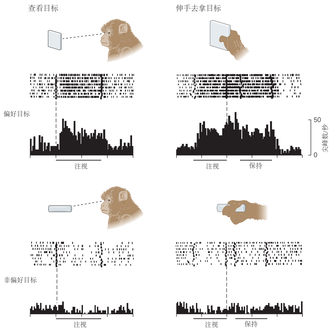
图 25.2.7: 顶内前皮层的神经元对特定的形状有选择性的响应。这里显示的神经元对矩形是有选择性的，无论是观察物体还是伸手去够。无论哪种情况，神经元都对圆柱体没有响应。
