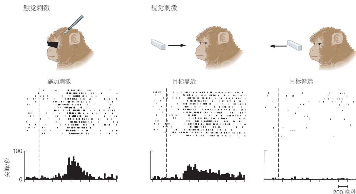
图 25.2.8: 猴子顶内皮层腹侧的双模态神经元对视觉和触觉刺激都有响应。这里显示的神经元对猴子头部的触觉刺激或朝向头部的视觉刺激做出响应，但对远离头部的相同刺激没有响应。
