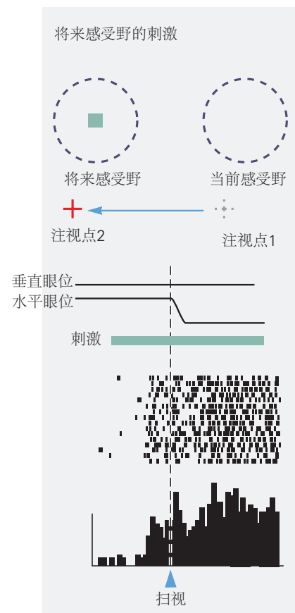
图 25.1.3: 重新映射猴子顶叶皮层视觉神经元的感受野与眼跳 [224] 。A. 左：猴子注视点，并且细胞对当前感受野中突然出现的与任务无关的刺激做出响应。连续试验在刺激出现时同步。右图：猴子看着注视点 1，细胞对未来感受野中闪现的刺激没有响应。B. 猴子从 注视点 1 到 注视点 2 进行眼跳，这会将细胞的感受野带到未来感受野中的刺激上。现在细胞甚至在眼跳开始之前就开始放电，这意味着扫视规划的伴随发送重新映射了细胞响应的视网膜区域。
