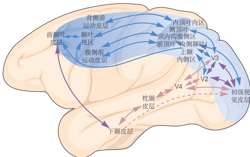
图 25.2.6: 动作视觉处理的通路。背侧视觉通路（蓝色）延伸到后顶叶皮层，然后延伸到额叶皮层。腹侧视觉通路（粉红色）见第 24 章。从下颞皮层到前额叶皮层有双向投射。
