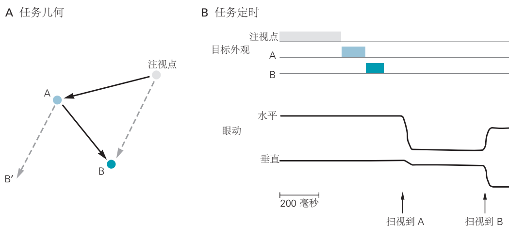
图 25.1.2: 双步任务说明大脑如何在眼跳期间稳定图像。A. 受试者首先注视一个消失的注视点，然后 2 个眼跳目标 A 和 B 依次出现和消失，然后受试者才能进行眼跳。第一个眼跳（目标 A）很简单。视网膜向量（注视点 \rightarrow A）和眼跳向量相同。第一次眼跳后，被试正在看 A，视网膜向量为 A \rightarrow B' ，但猴子必须进行一次眼跳，向量为 A \rightarrow B 。大脑必须调整视网膜向量以补偿第一个眼跳。B. 时序。上面的记录显示目标出现的时间（彩色条）。
