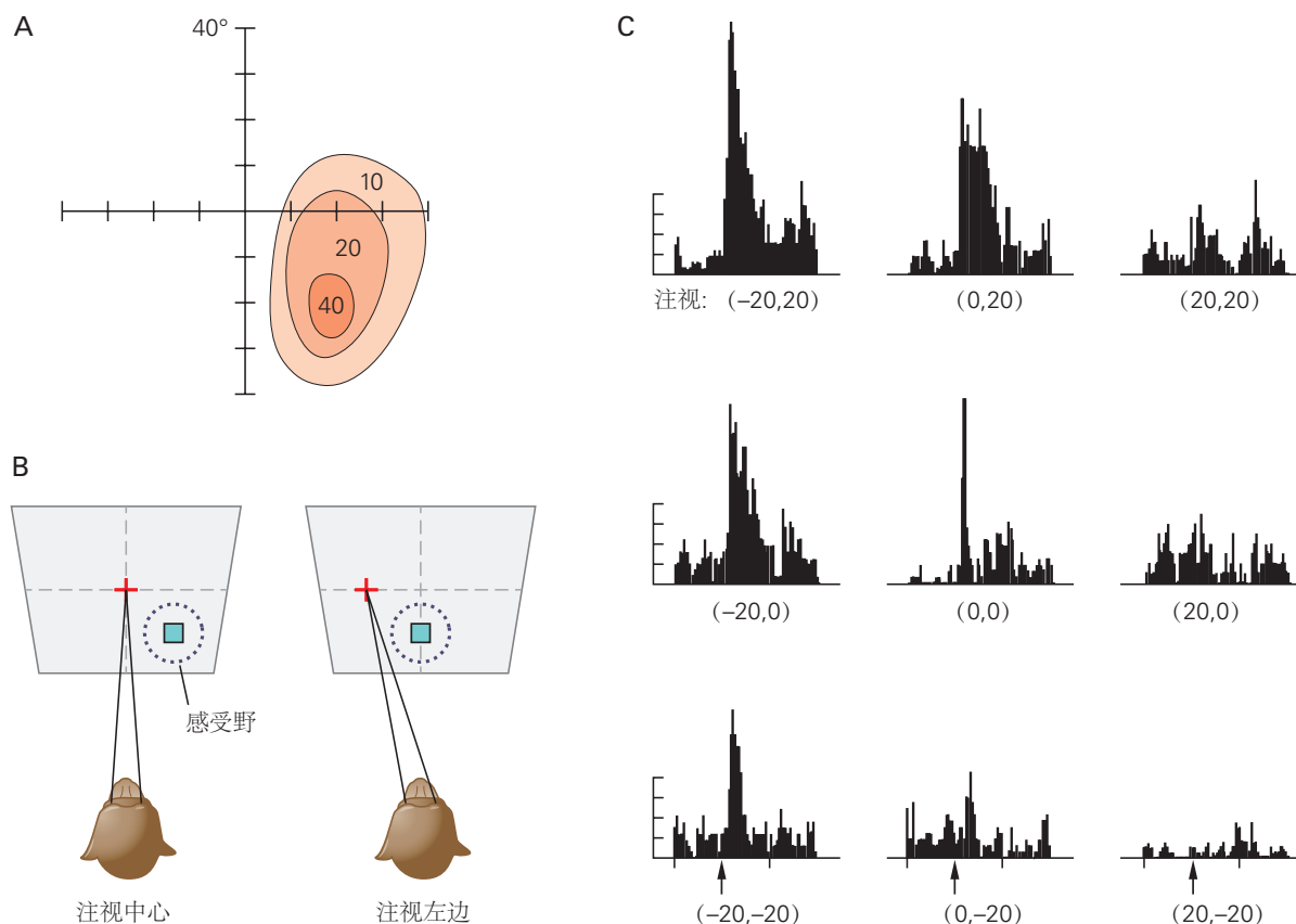
图 25.1.6: 眼球在眼眶中的位置会影响具有视网膜拓扑感受野的顶叶视觉神经元的响应。A. 相对于中央凹的感受野。等高线图表示不同空间位置的脉冲率。数字表示每个等高线在最大位置的每秒脉冲率。B. 感受野随眼睛在空间移动。在左图，猴子正在注视屏幕的中心。在右图，同一只猴子注视着中心左侧 20^\circ 。对于 C 中的记录，刺激（蓝色方块）始终呈现在感受野的中心。C. 在感受野的最佳位置对刺激的响应随着眼睛在眼眶中的位置而变化，从猴子注视 (-20^\circ, 20^\circ) 时的最大值到猴子注视 (20^\circ, -20^\circ) 时的最小值。箭头表示刺激闪光的开始。试验时间为 1.5 秒；纵坐标中每一格表示 25 个脉冲 [227] 。
