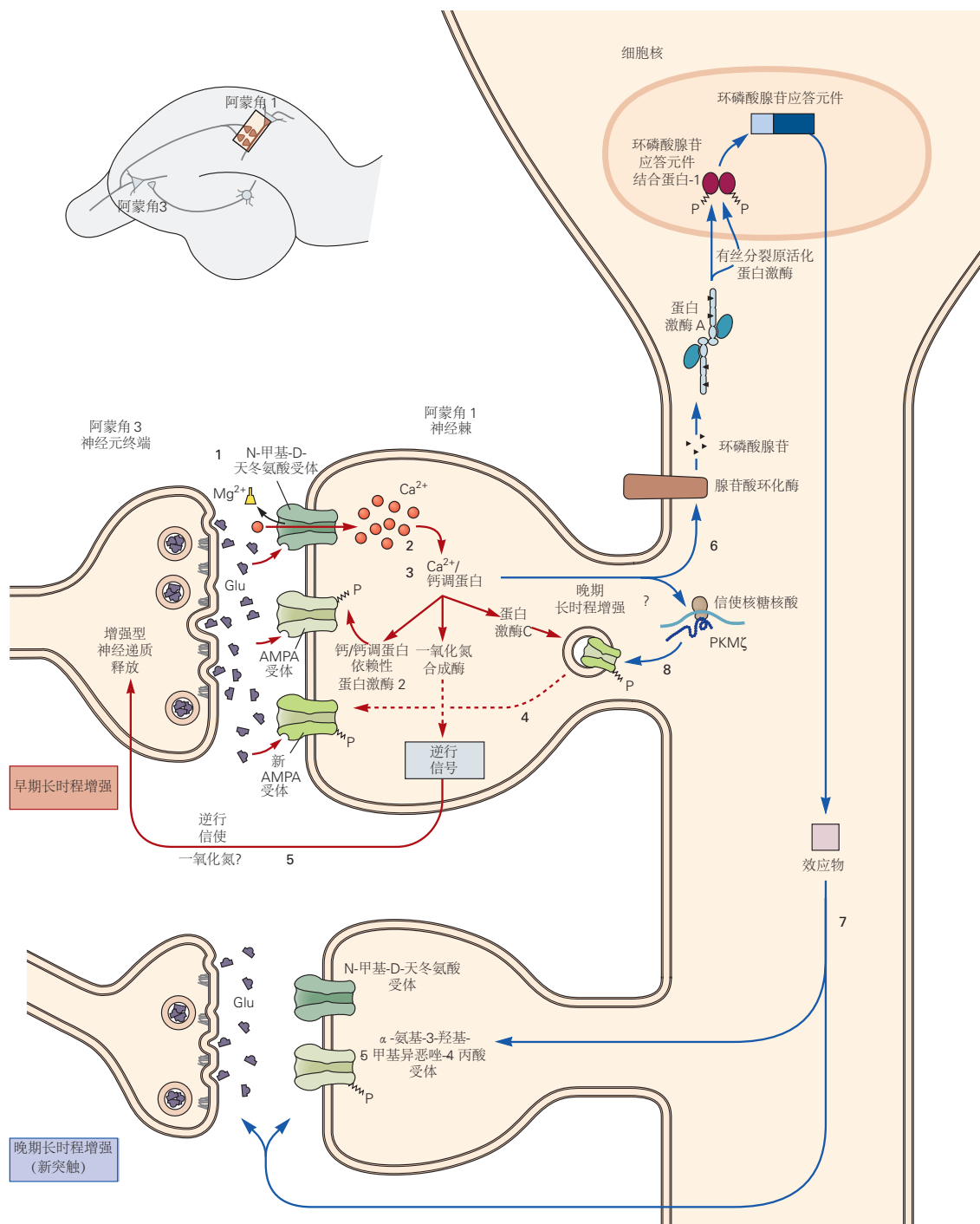
图 54.1.3: 在谢弗侧支突触诱导长时程增强的模型。一次高频强直刺激会诱发早期长时程增强。突触后膜的大量去极化（由 AMPA 受体的强烈激活引起）减轻了 NMDA 的 Mg^{2+} 阻断受体通道（1），允许 Ca^{2+} 、 Na^+ 和 K^+ 流过这些通道。由此导致的树突棘中 Ca^{2+} 的增加（2）触发钙依赖性激酶（3）（钙/钙调蛋白依赖性蛋白激酶 2 和蛋白激酶 C）导致长时程增强的诱导。在诱导长时程增强期间激活的第二信使级联对突触传递有 2 个主要影响。通过激活蛋白激酶 C 进行的磷酸化增强了通过 AMPA 受体通道的电流，部分原因是导致新受体插入脊柱突触（4）。此外，突触后细胞释放逆行信使，如一氧化氮，激活突触前末梢的蛋白激酶以增强随后的递质释放（5）。反复发生的强直刺激会诱发晚期长时程增强。 Ca^{2+} 内流的持续增加会募集腺苷酸环化酶（6），后者会生成可激活蛋白激酶 A 的环磷酸腺苷。这导致有丝分裂原活化蛋白激酶的激活，它转移到细胞核，在那里磷酸化环磷酸腺苷应答元件结合蛋白-1。环磷酸腺苷应答元件结合蛋白-1 反过来激活目标（包含环磷酸腺苷应答元件启动子）的转录，这些目标被认为会导致新突触连接的生长（7）。重复刺激还会激活编码蛋白激酶 Mζ 的信使核糖核酸的翻译，蛋白激酶 Mζ 是蛋白激酶 C 的组成型活性亚型（8）。这导致突触后膜中 AMPA 受体数量的长期增加。
