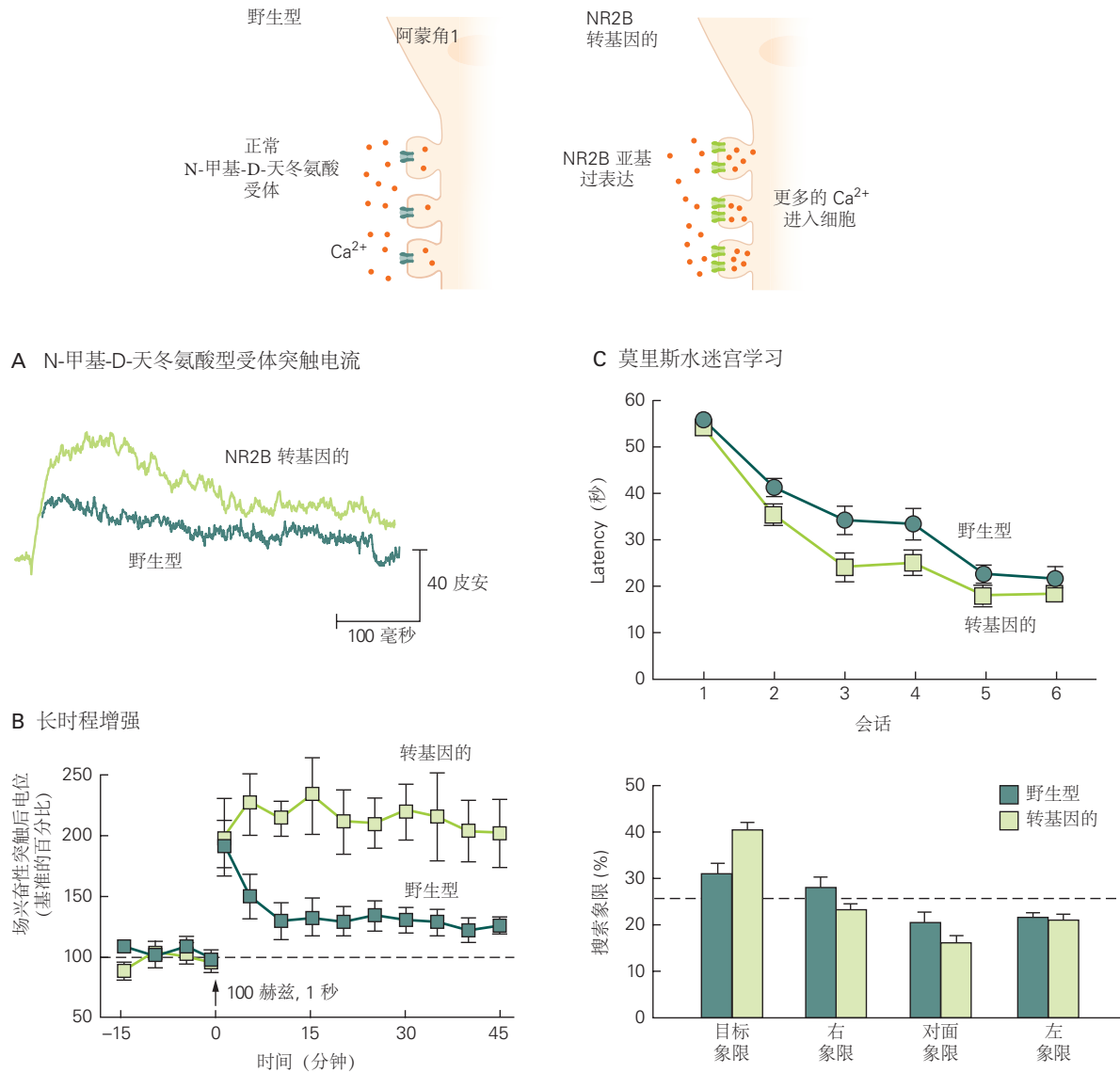
图 54.1.8: 过度表达 NMDA 谷氨酸受体亚基的小鼠的学习和记得到增强。 A. NMDA 受体响应谷氨酸的短暂脉冲而产生的电流振幅增强, 其在海马体神经元中的时程延长从含有转基因的小鼠中获得, 与野生型小鼠相比, 该转基因表达更高水平的受体 NR2B 亚基。 B. 强直刺激 谢弗侧支突触产生的长时程增强在转基因小鼠中比在野生型小鼠中更大。 C. 转基因小鼠的空间学习得到增强 (上图)。转基因小鼠在莫里斯水迷宫中的学习速度 (减少寻找隐藏平台的时间, 或逃避延迟) 比野生型小鼠更快。转基因小鼠的空间记忆也得到增强 (下图)。在探测试验中, 转基因小鼠比野生型小鼠在目标象限中停留的时间更长, 该象限之前包含隐藏平台。
