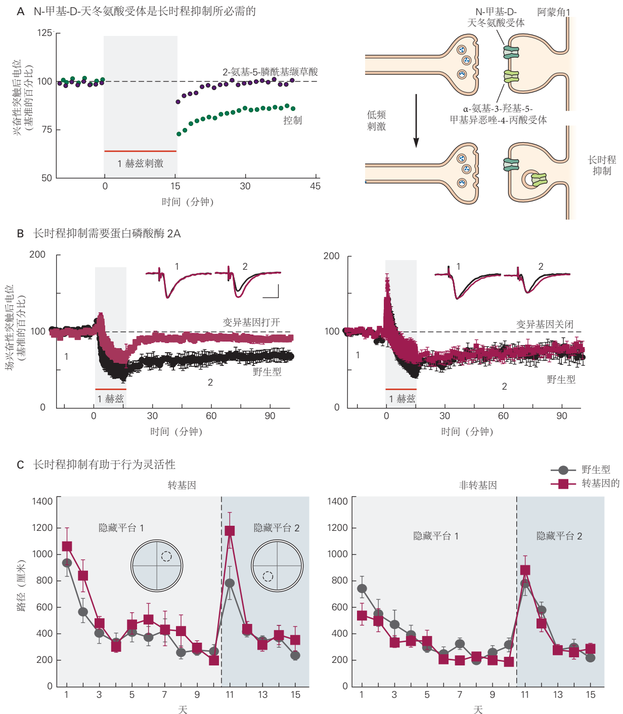
图 54.2.1: 突触传递的长时程抑制需要 NMDA 受体和磷酸酶活性。 A. 对谢弗侧支纤维的长时间低频刺激 (1 赫兹, 15 分钟) 会导致海马体阿蒙角 1 区兴奋性突触后电位场的大小长期下降, 这种下降比刺激持续时间更长 (控制)。当 AMPA 受体通过内存作用从突触后膜移除时, 会发生长时程抑制; 当 NMDA 受体被药物 2-氨基-5-噻吩基羧酸阻断时, 它被阻断 [517] 。B. 长时程抑制需要蛋白质去磷酸化。该图比较了野生型小鼠和表达抑制磷酸酶 2A 的蛋白质的转基因小鼠海马体阿蒙角 1 区的长时程抑制。转基因表达受 tTA 系统控制。在没有多西环素的情况下, 表达磷酸酶抑制剂, 并抑制长时程抑制的诱导 (左图)。当通过施用多西环素关闭磷酸酶抑制剂的表达时, 会诱导正常大小的长时程抑制 (右图)。C. 抑制磷酸酶 2A 会降低行为灵活性。表达磷酸酶抑制剂的转基因小鼠以与野生型小鼠相同的速度 (第 1-10 天) 学习莫里斯迷宫中水下平台的位置。因此, 长时程抑制不是学习初始平台位置所必需的。在第 10 天结束时, 平台被移动到一个新的隐藏位置并重新测试小鼠 (第 11-15 天)。现在, 转基因小鼠在重新测试的第一天 (第 11 天) 要走更长的路才能找到平台, 这表明学习受损 (灵活性降低)。当用多西环素关闭转基因表达时, 转基因小鼠在测试的所有阶段都表现出正常的学习能力 [518] 。
