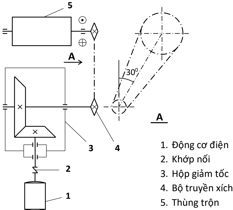
Hình 1: Sơ đồ động
