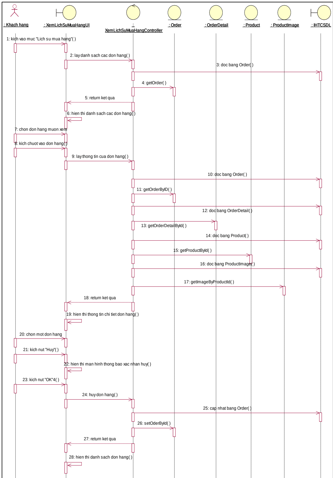
Hình 2. 24 Biểu đồ trình tự use case xem lịch sử mua hàng
