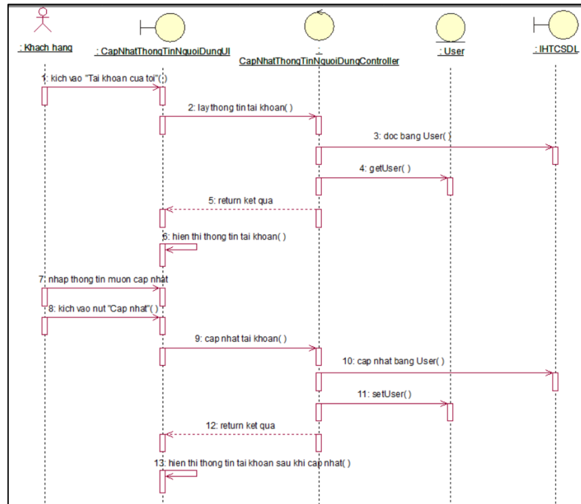
Hình 2. 13 Biểu đồ trình tự use case cập nhật thông tin người dùng
