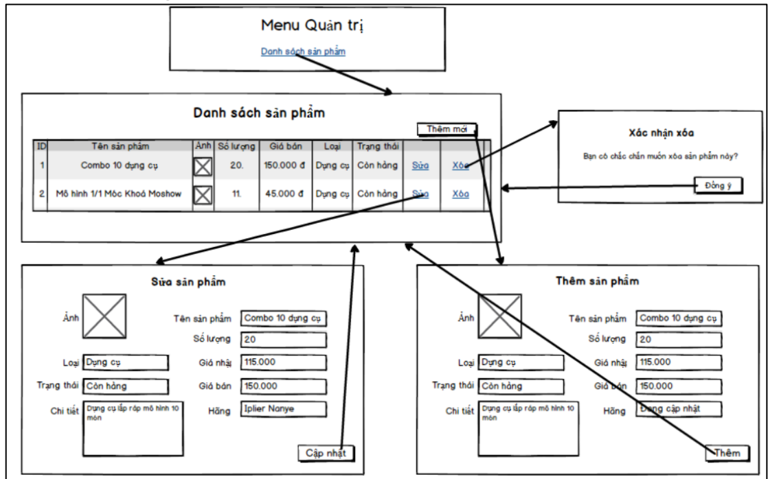
Hình 2. 44 Hình dung màn hình use case quản lý sản phẩm
