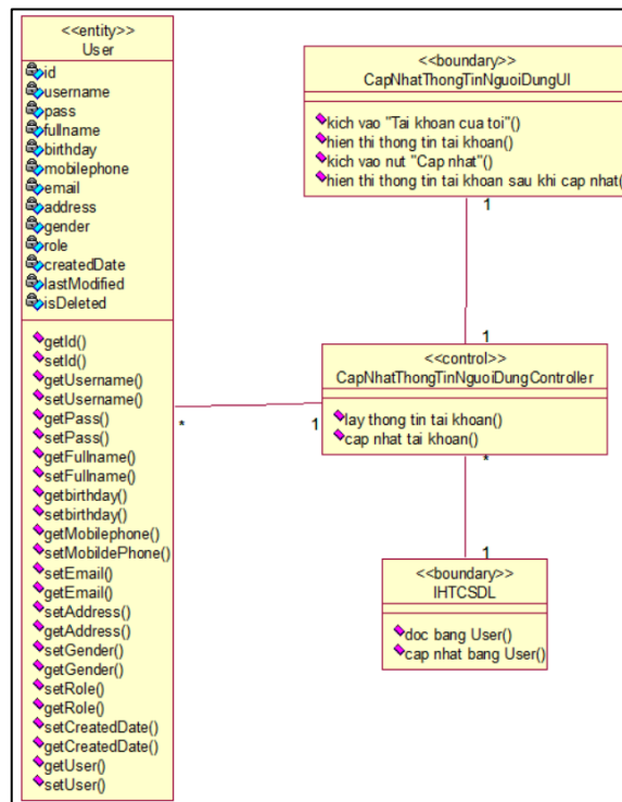
Hình 2. 14 Biểu đồ VOPC use case cập nhật thông tin người dùng
