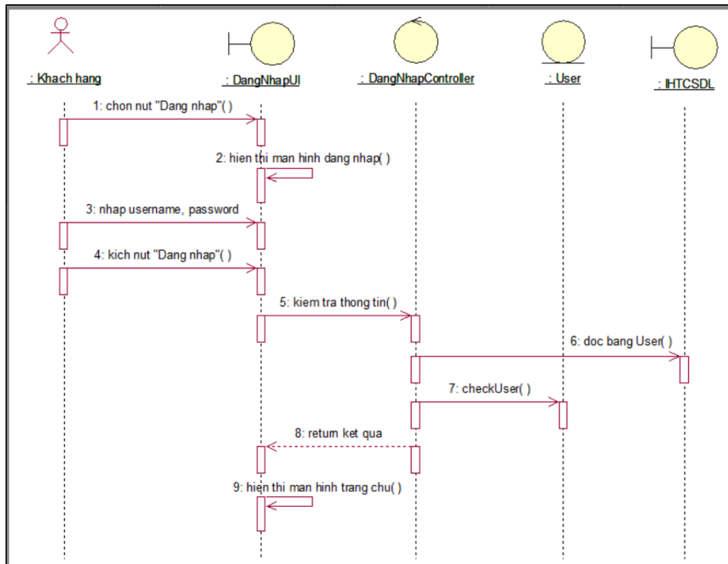
Hình 2. 9 Biểu đồ trình tự use case đăng nhập
