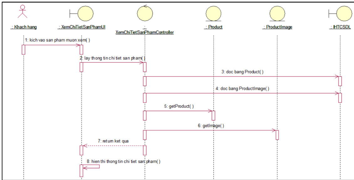
Hình 2. 17 Biểu đồ trình tự use case xem chi tiết sản phẩm
