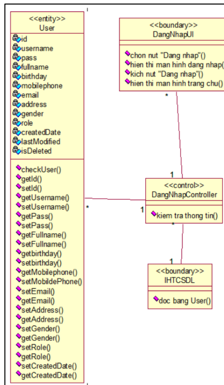
Hình 2. 10 Biểu đồ VOPC use case đăng nhập
