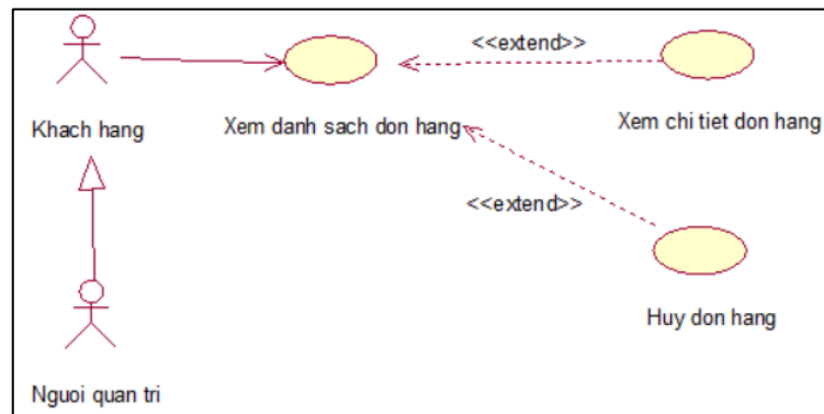
Hình 2. 3 Phân rã use case xem danh sách lịch sử mua hàng
