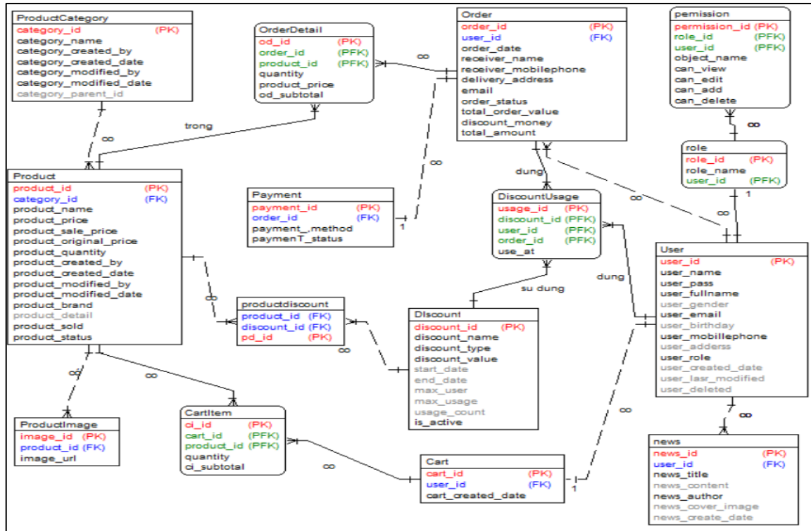
Hình 2. 50 Biểu đồ thực thể liên kết mức Logic
