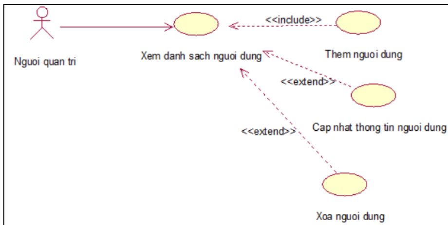
Hình 2. 7 Phân rã use case quản lý người dùng
