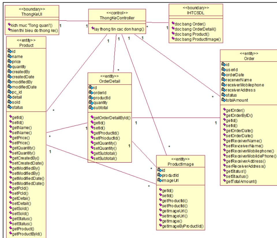
Hình 2. 32 Biểu đồ VOPC use case thống kê
