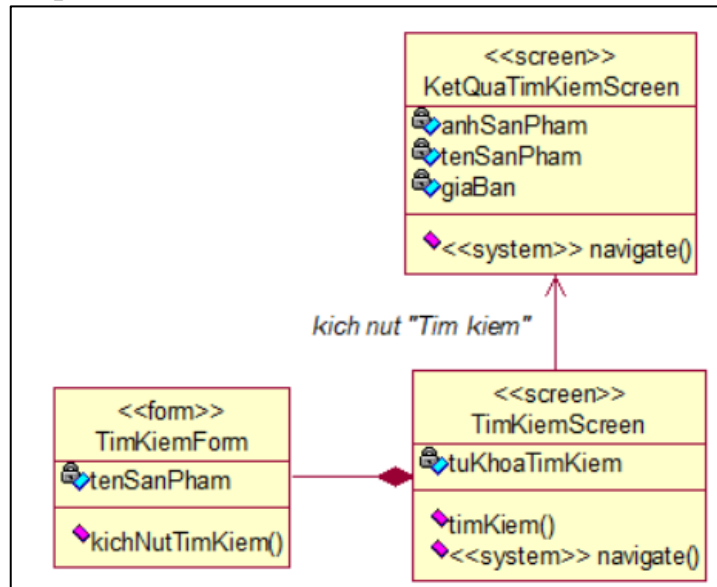
Hình 2. 36 Biểu đồ lớp phân tích use case tìm kiếm sản phẩm
