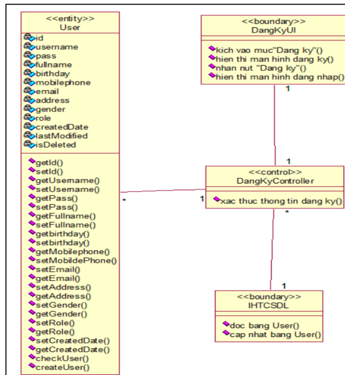
Hình 2. 12 Biểu đồ VOPC use case đăng ký
