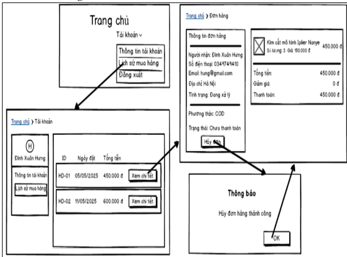
Hình 2. 41 Hình dung màn hình use case xem chi tiết đơn hàng
