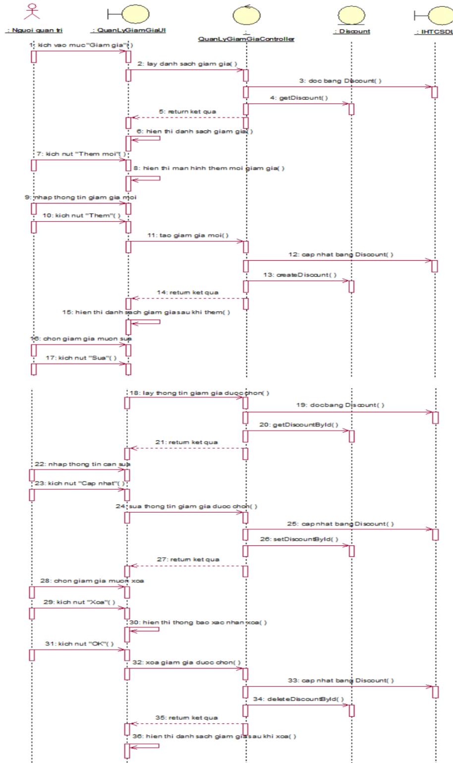
Hình 2. 33 Biểu đồ trình tự use case quản lý giảm giá
