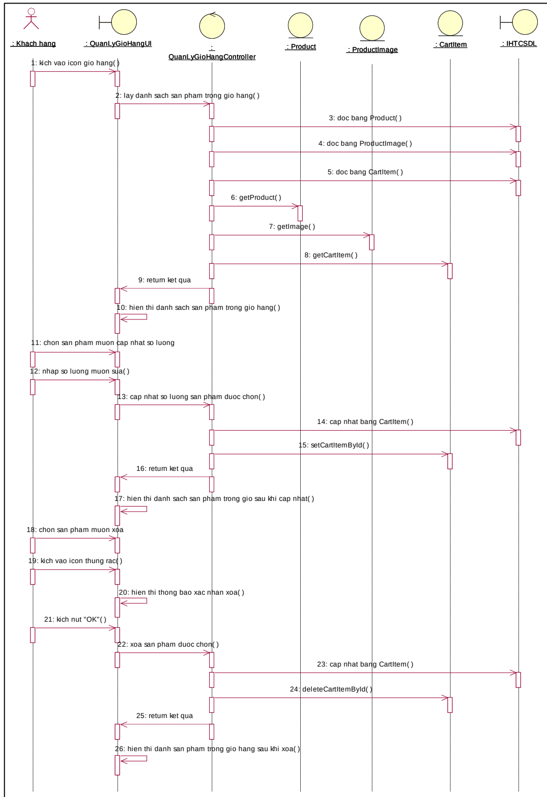
Hình 2. 21 Biểu đồ trình tự use case quản lý giỏ hàng
