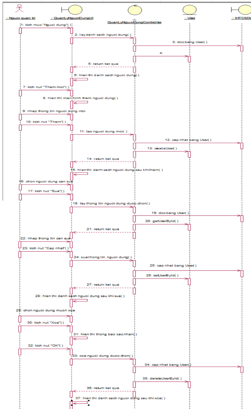
Hình 2. 30 Biểu đồ trình tự use case quản lý người dùng
