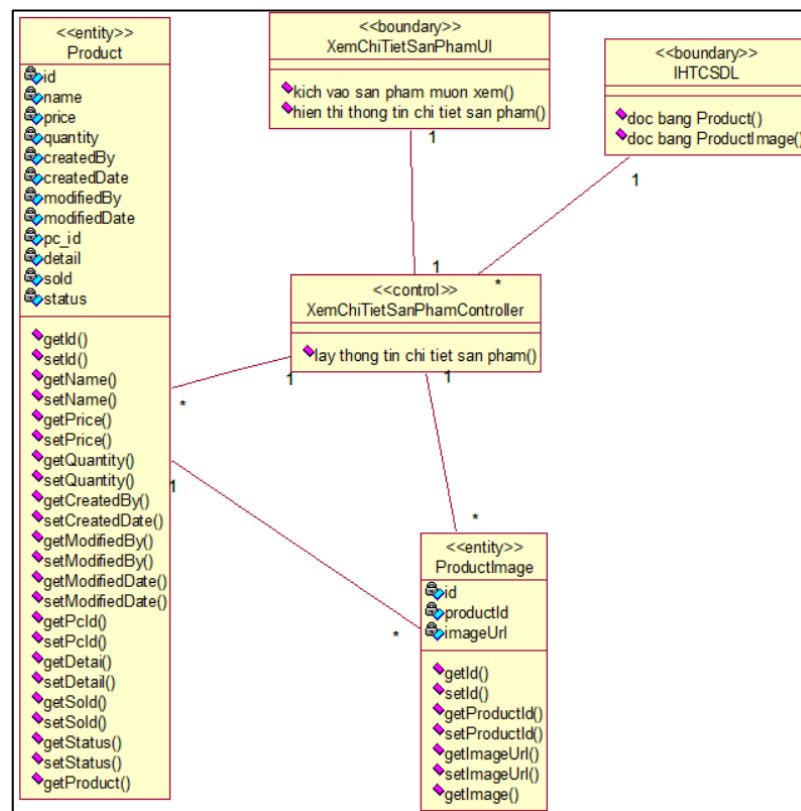
Hình 2. 18 Biểu đồ VOPC use case xem chi tiết sản phẩm
