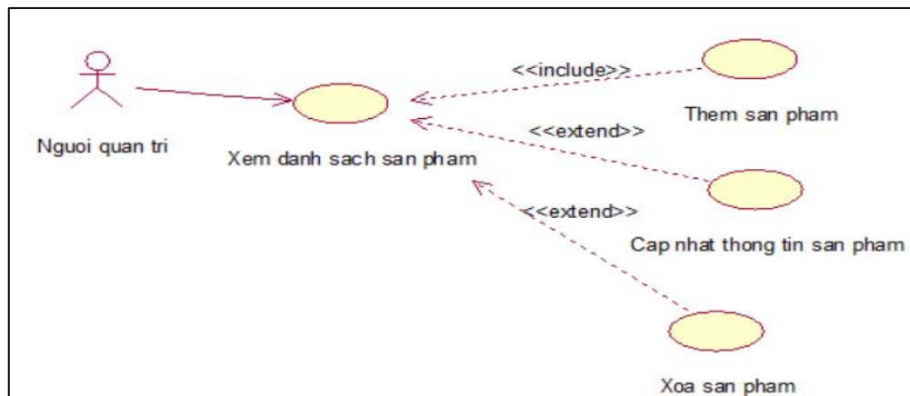
Hình 2. 4 Phân rã use case quản lý sản phẩm
