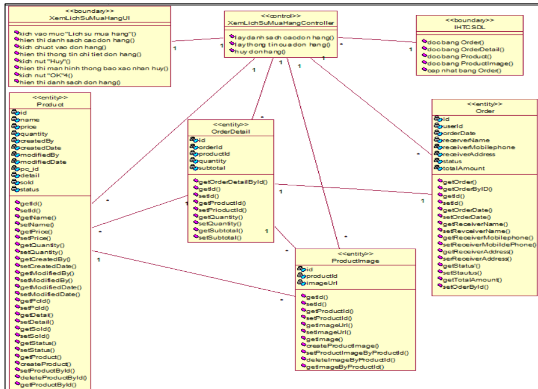
Hình 2. 23 Biểu đồ VOPC use case xem lịch sử mua hàng
