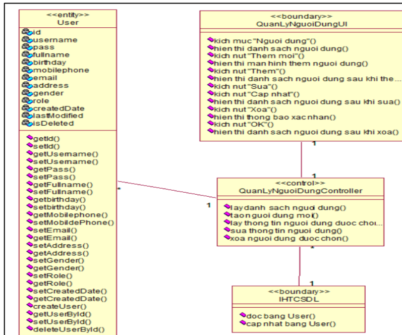
Hình 2. 29 Biểu đồ VOPC use case quản lý người dùng
