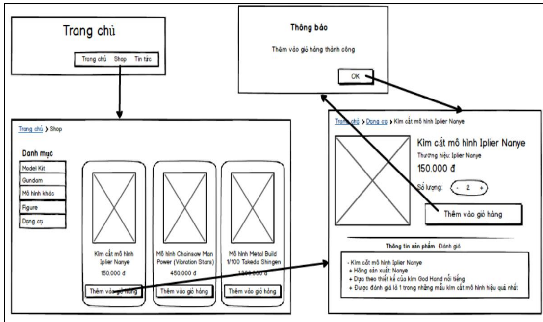
Hình 2. 38 Hình dung màn hình use case thêm sản phẩm vào giỏ hàng
