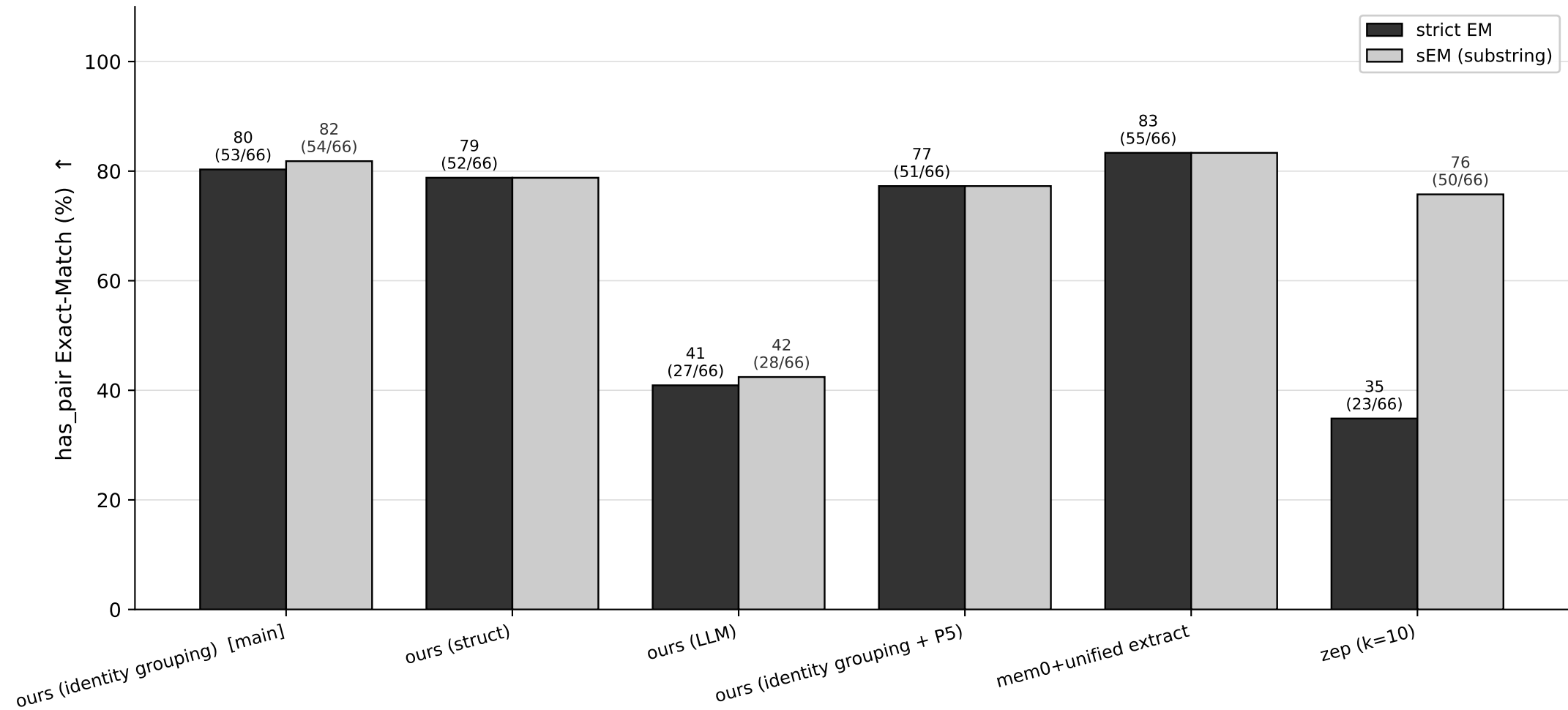
FC-SH 64k has_pair EM — all methods @ gpt-4.1-mini backbone (strict EM vs sEM)
