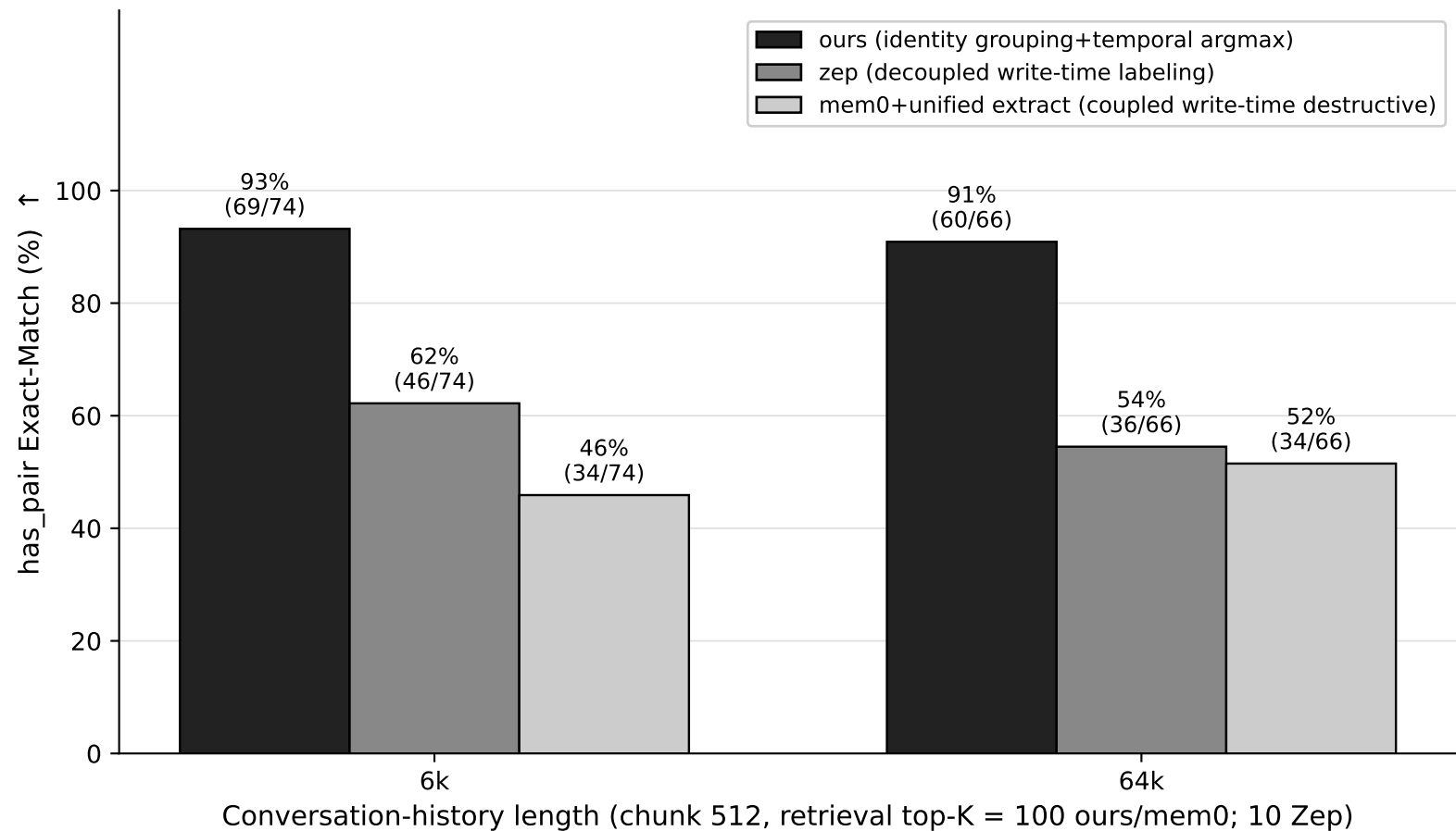
FC-SH has_pair EM — main comparison @ gpt-4o-mini backbone
