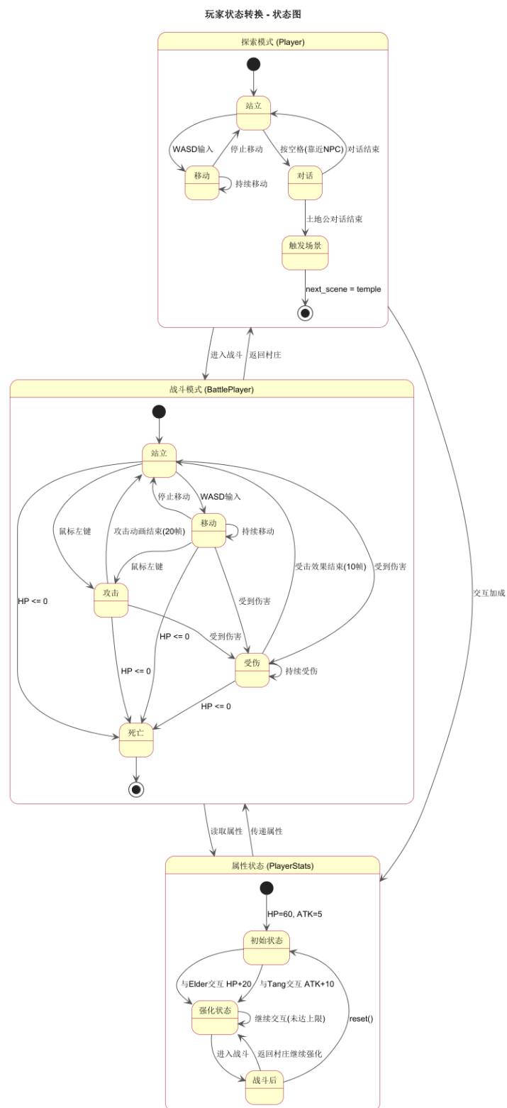
图 5: 玩家状态转换图
