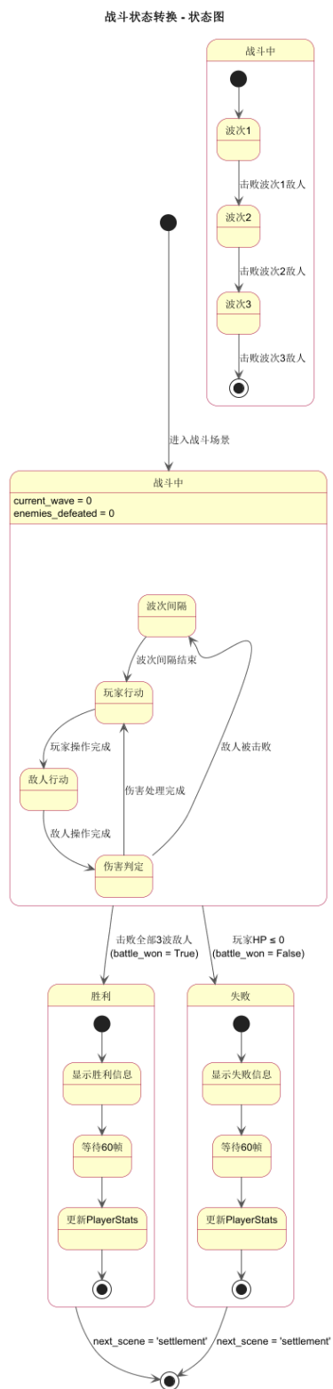
图 4: 战斗状态转换图
