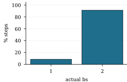
OpenVLA cfg=2
