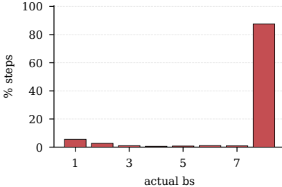
OpenVLA cfg=8
