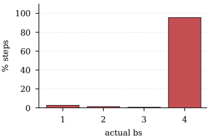
OpenVLA cfg=4
