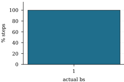
OpenVLA cfg=1
