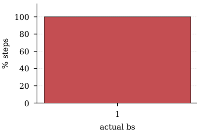
OpenVLA cfg=1
