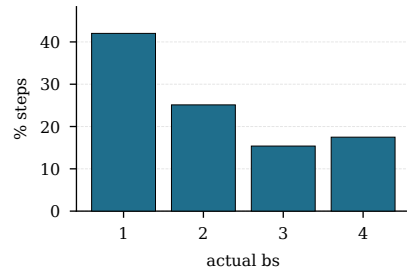
OpenVLA cfg=4
