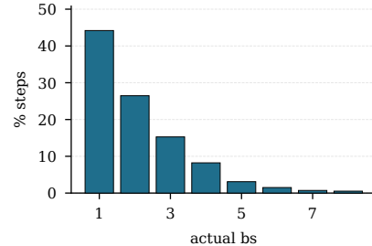
OpenVLA cfg=8
