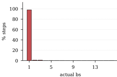
OpenVLA cfg=16
