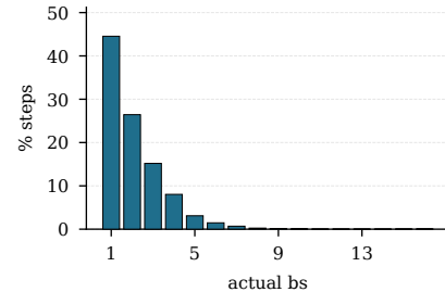
OpenVLA cfg=16
