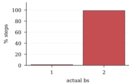
OpenVLA cfg=2
