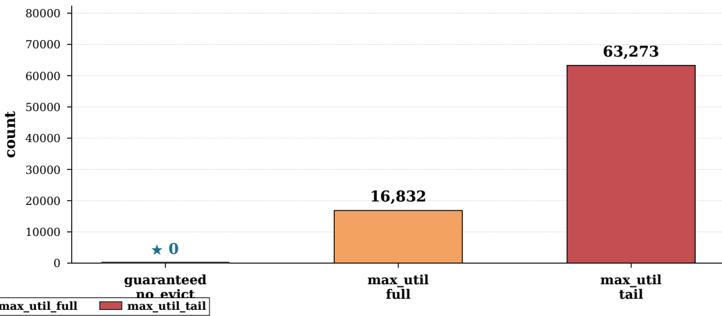
(d) Tokens recomputed (wasted work)
