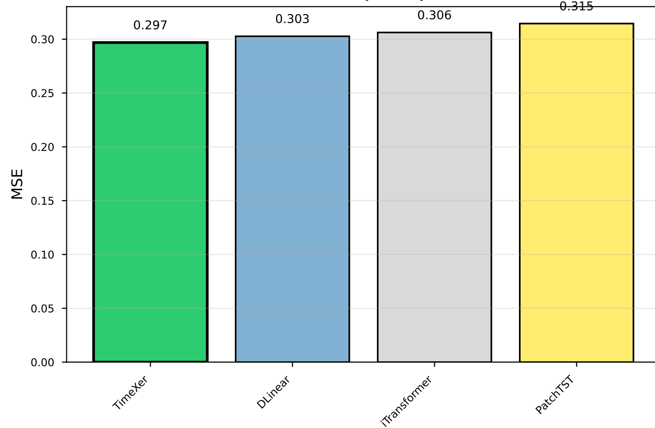
ETTm2 (H=96)
