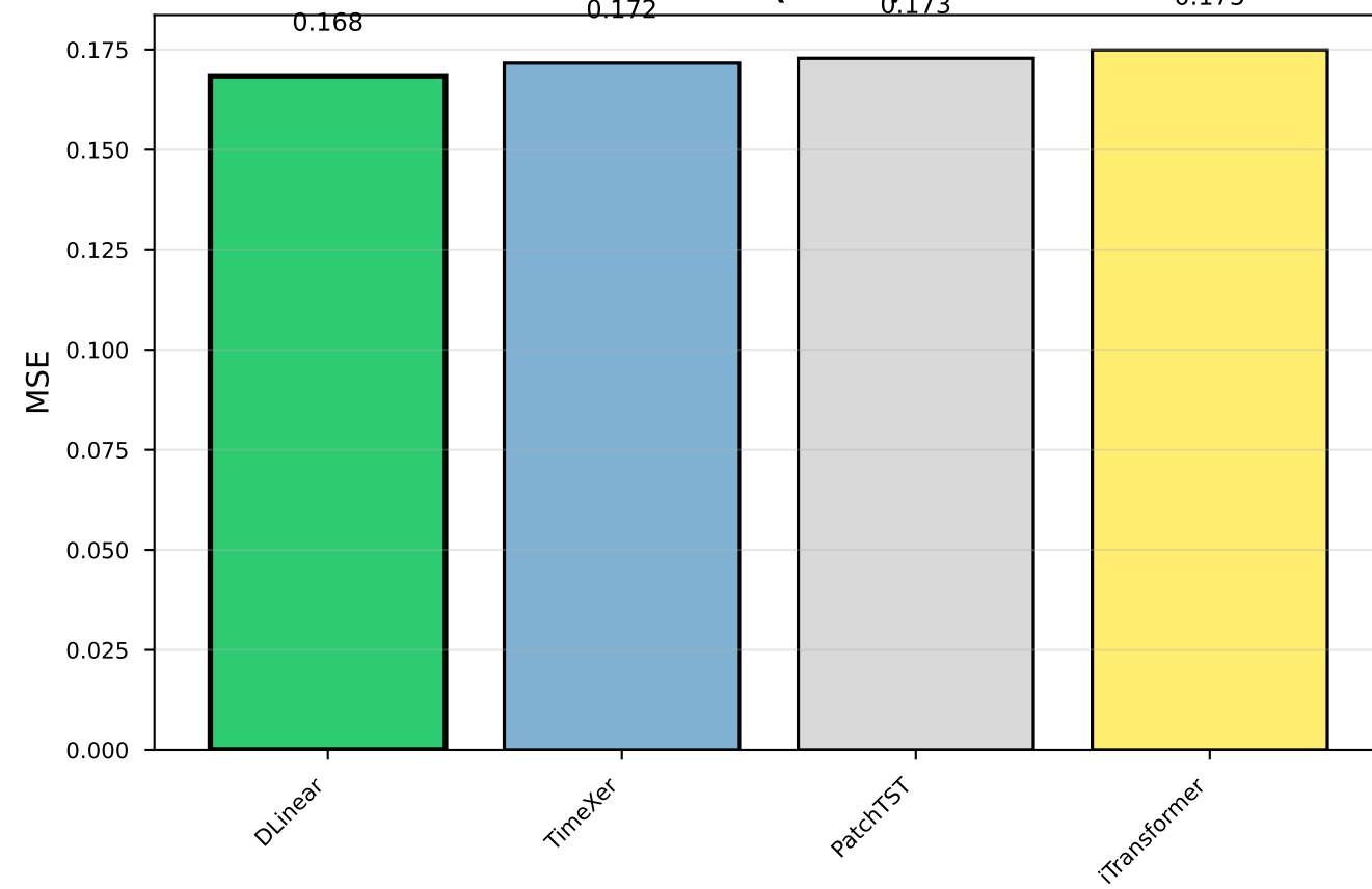
ETTm2 (H=96)
