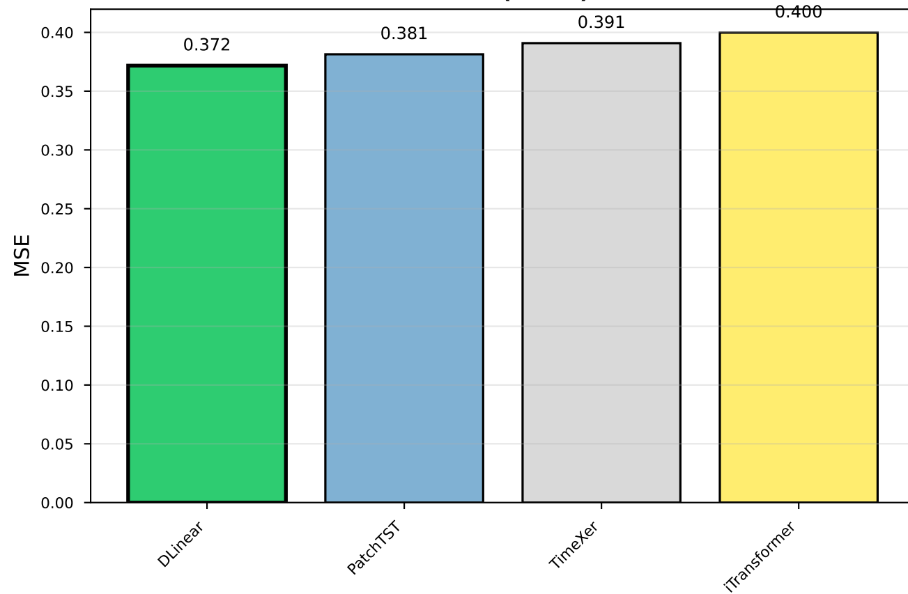
ETTm1 (H=96)
