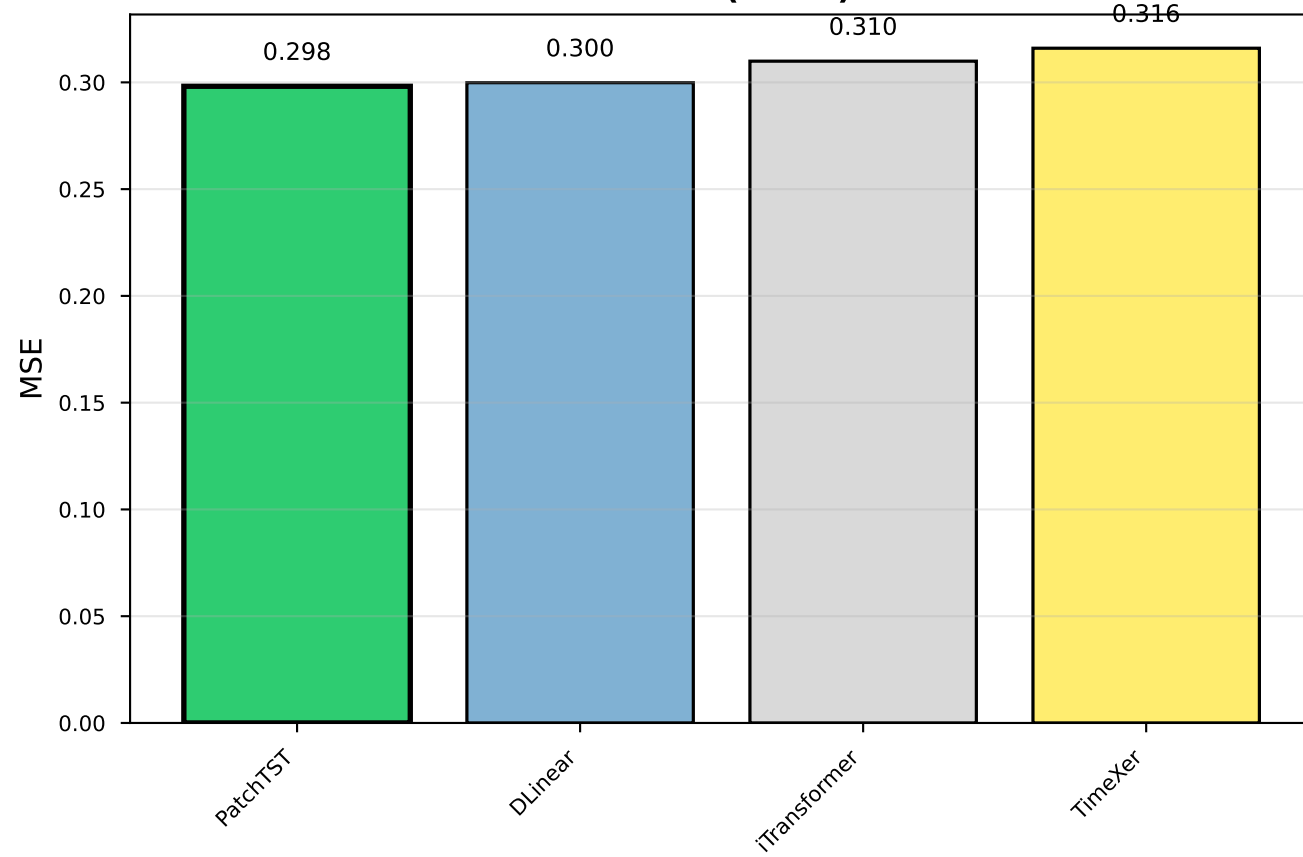
ETTm1 (H=96)
