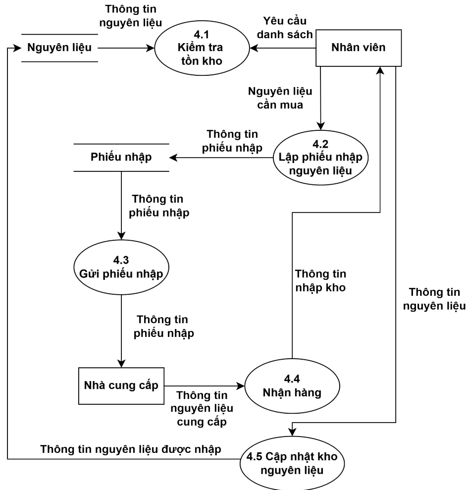
Hình 3.5. Sơ đồ DFD nhập hàng
