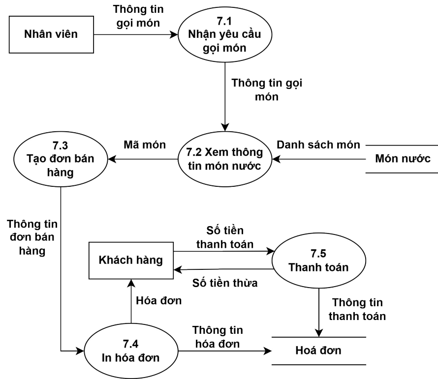
Hình 3.6. Sơ đồ DFD bán hàng
