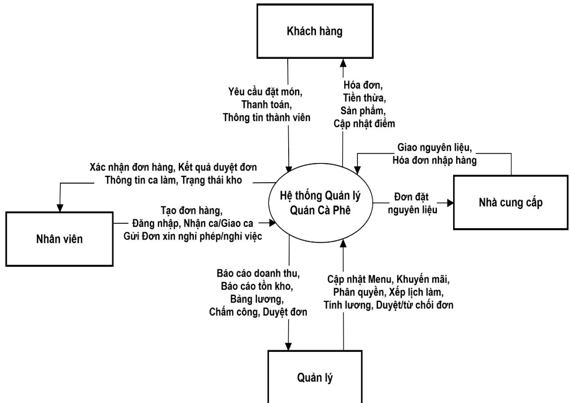
Hình 3.1. Sơ đồ DFD mức 0
