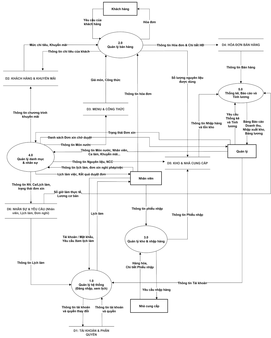
Hình 3.2. Sơ đồ DFD mức 1
