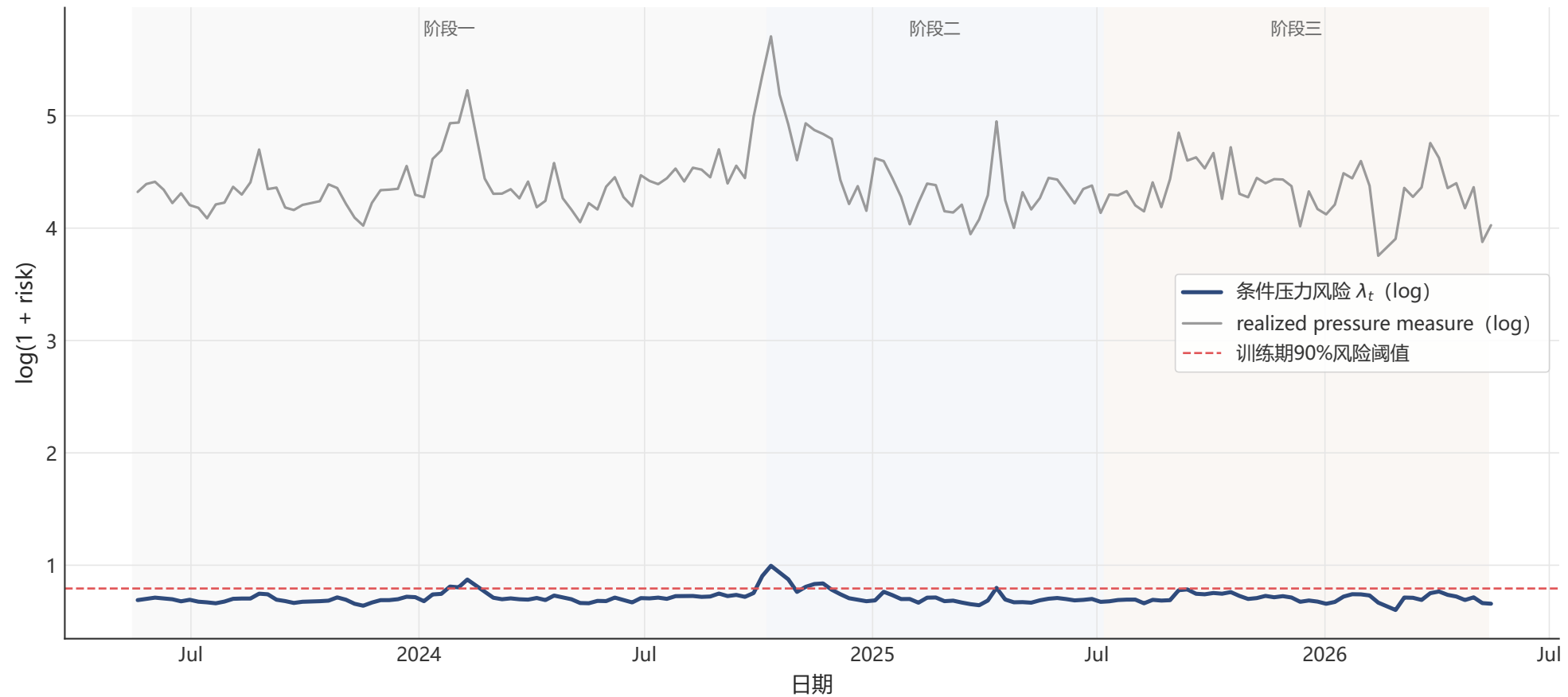
RGARCH-CARR-SK 条件压力风险路径
