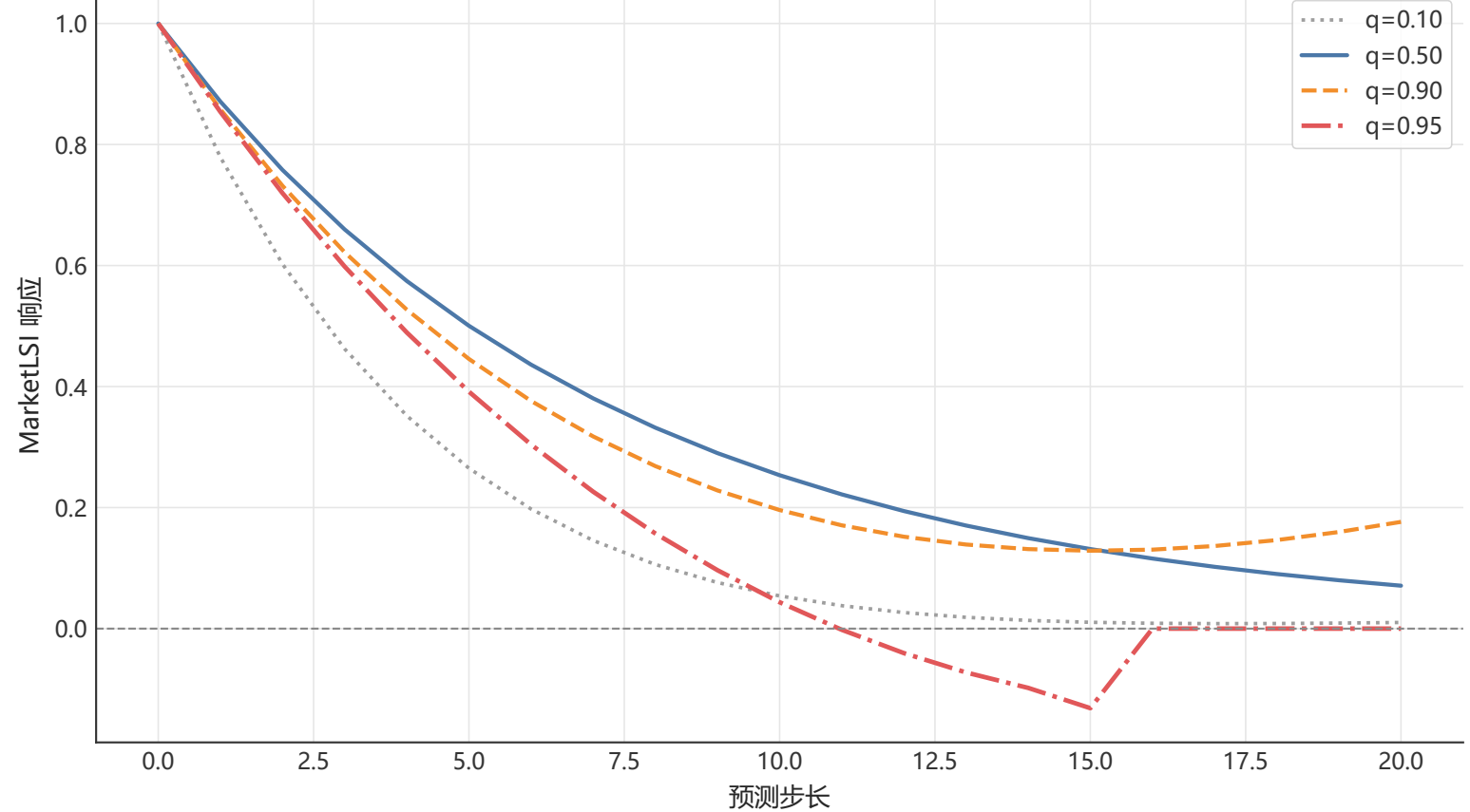
QVAR 尾部分位响应：MarketLSI shock
