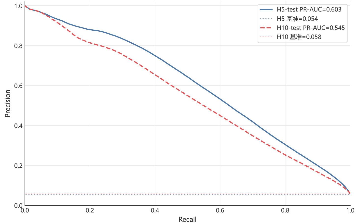
SMARTBoost 样本外 PR 曲线
